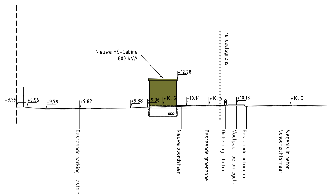
Terreinprofiel T1-Nieuwe toestand
