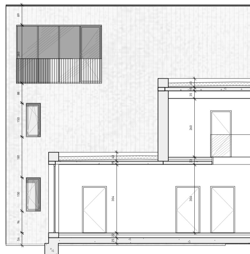
DOORSNEDE C
