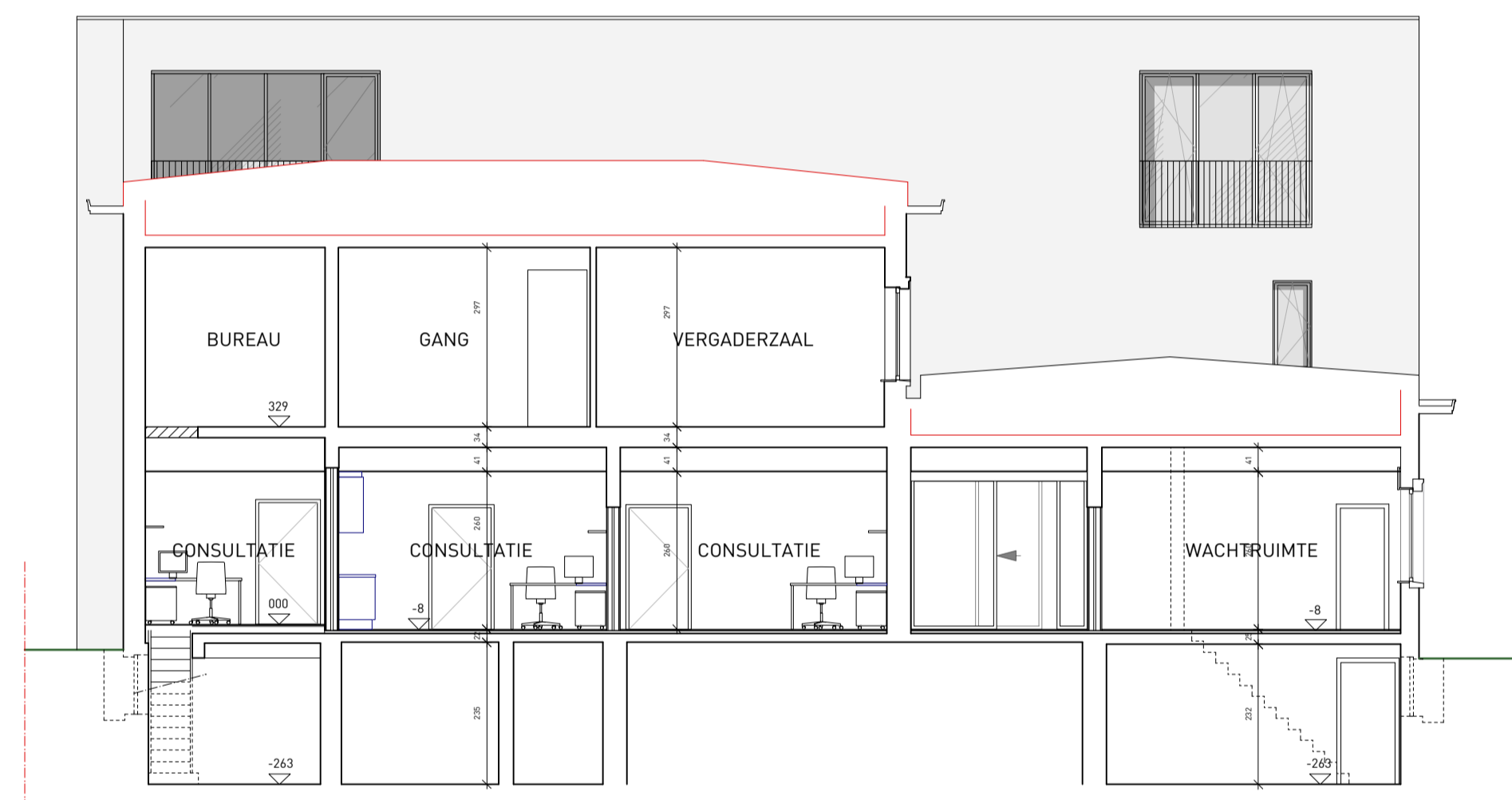
DOORSNEDE A
