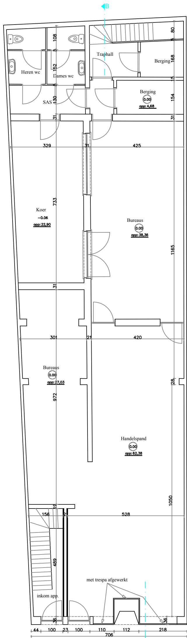
Gelijkvloers Bestaande toestand Schaal 1/100
