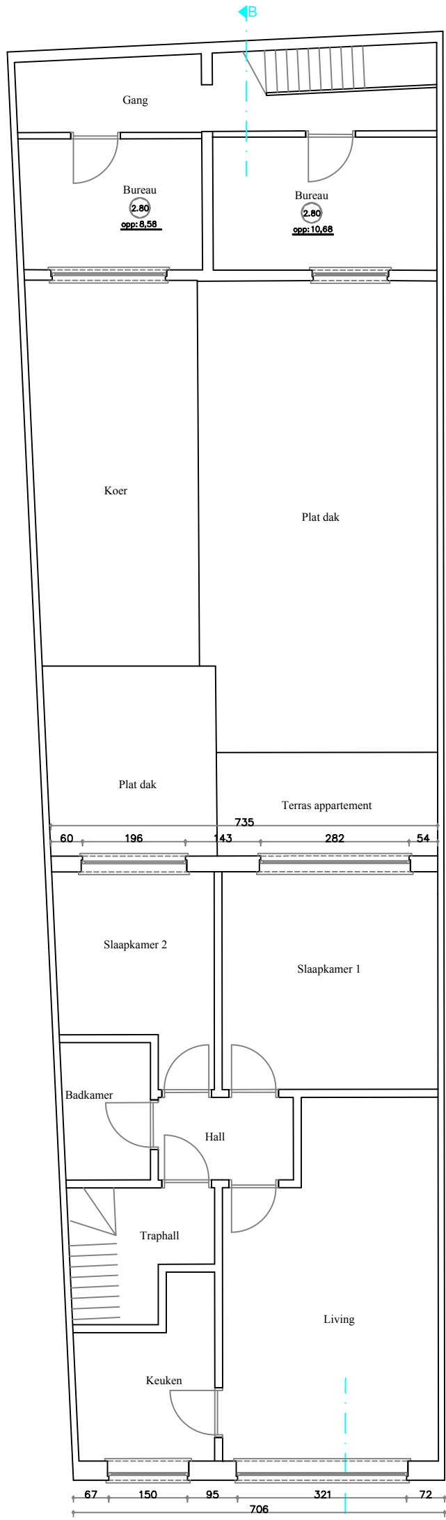
Eerste Verdieping Bestaande toestand Schaal 1/100
