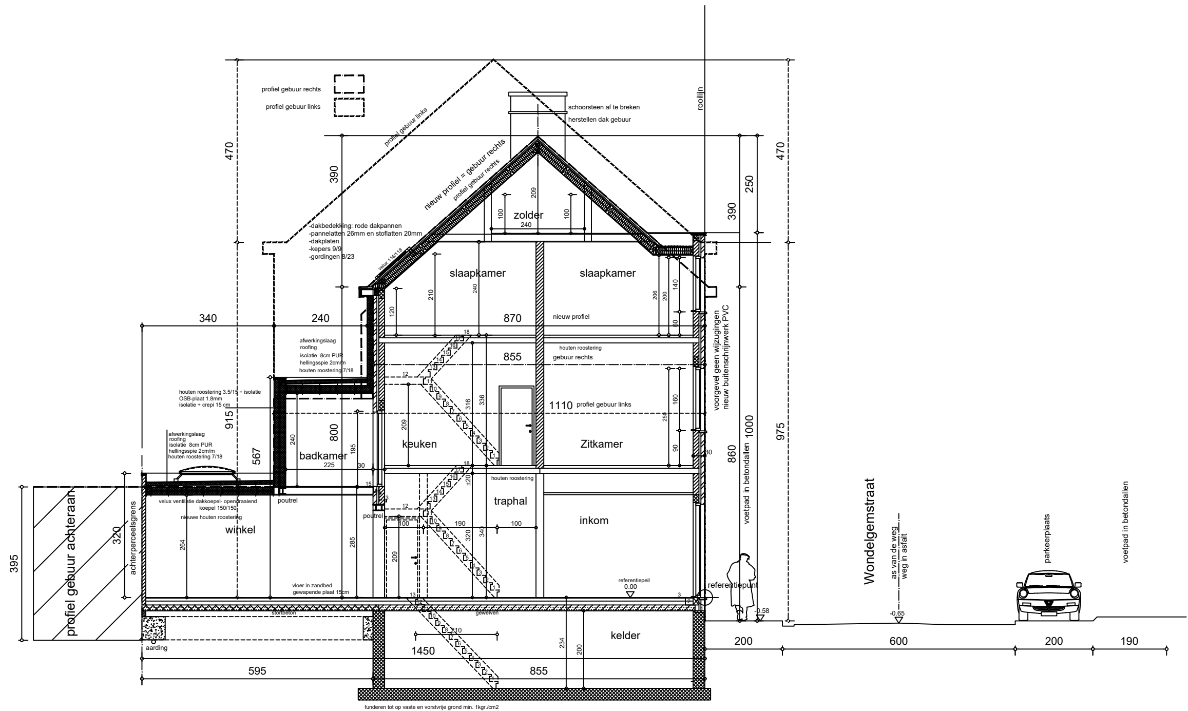
nieuwe toestand doorsnede aa / 1:100
