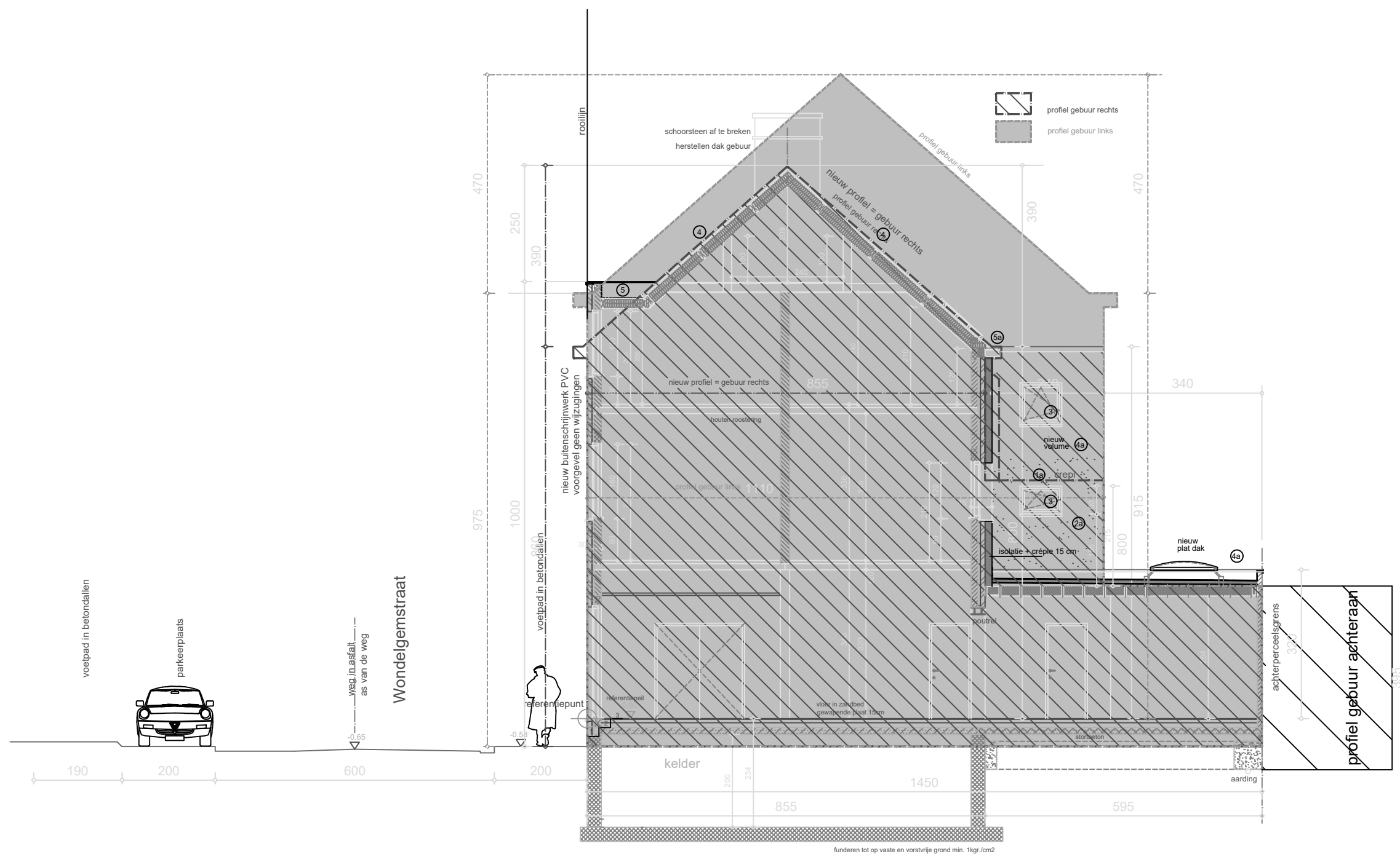
nieuwe toestand zijgevel rechts / 1:100
