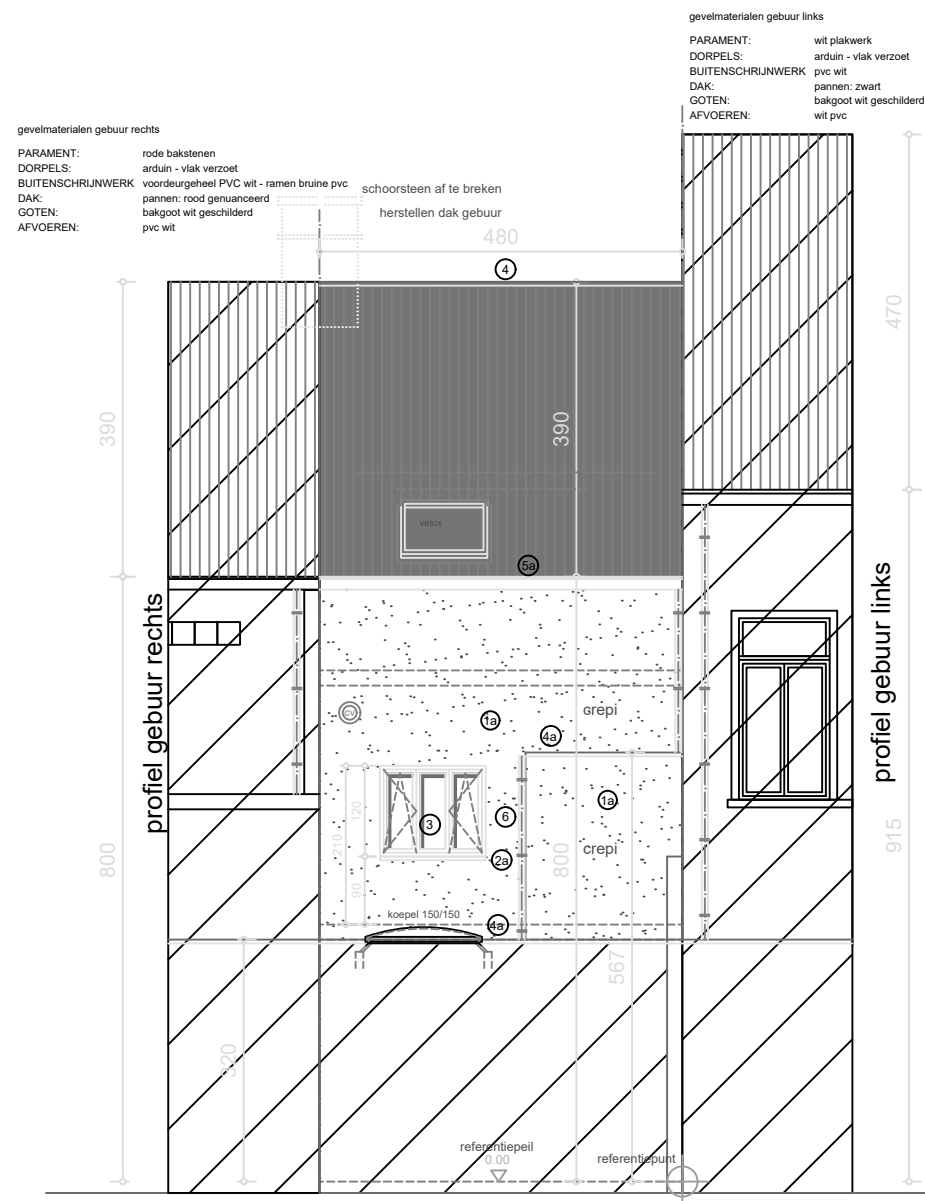
vergunde toestand achtergevel / 1:100
