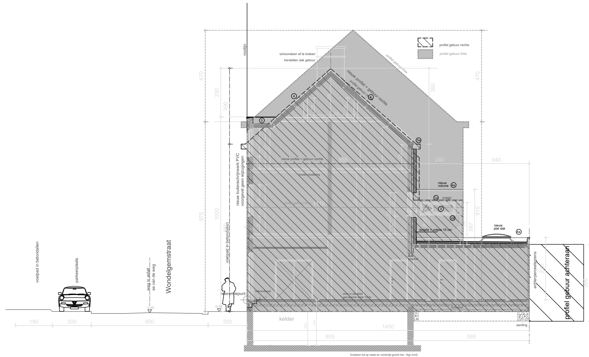
vergunde toestand zijgevel rechts / 1:100
