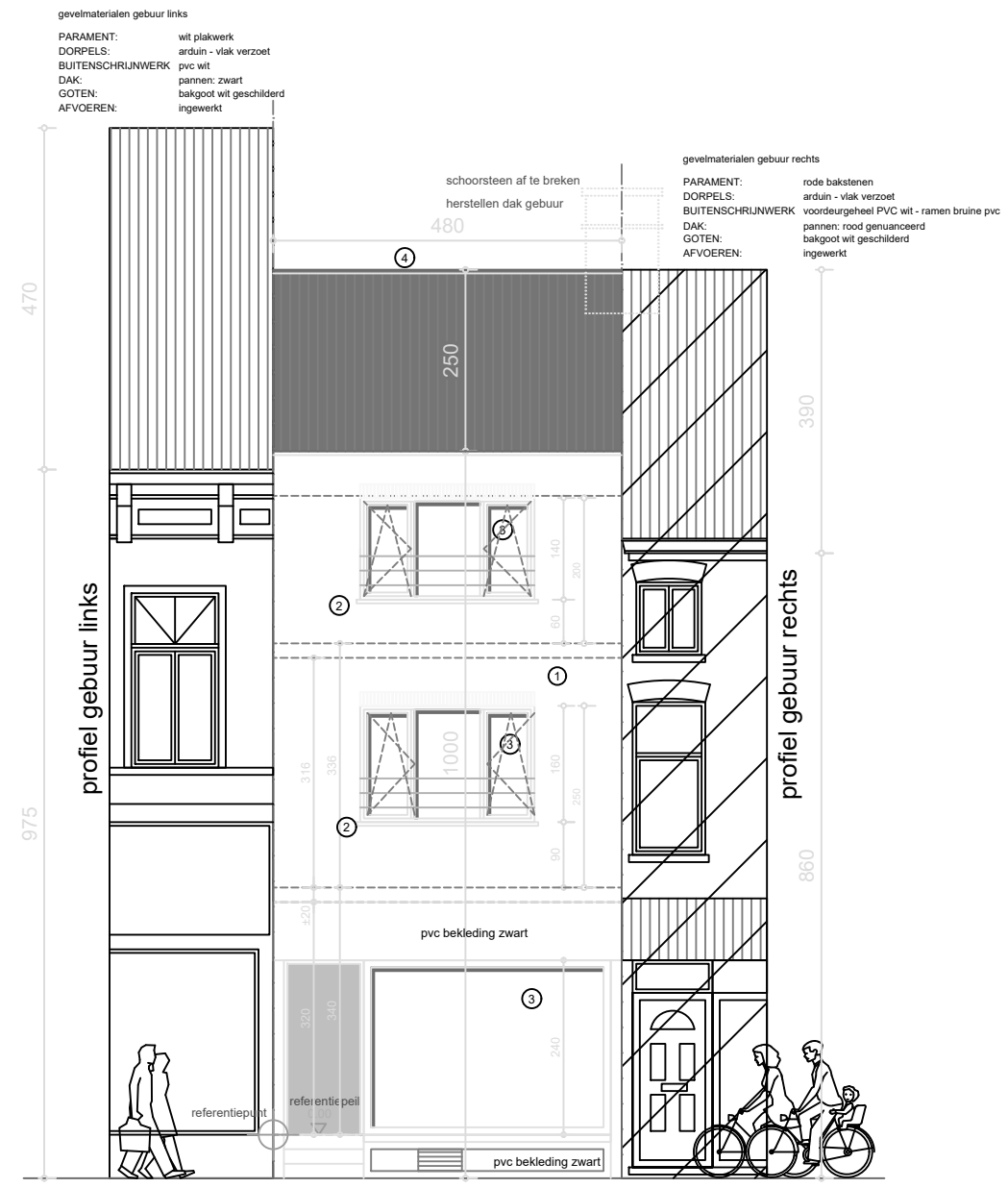
nieuwe toestand voorgevel / 1:100
