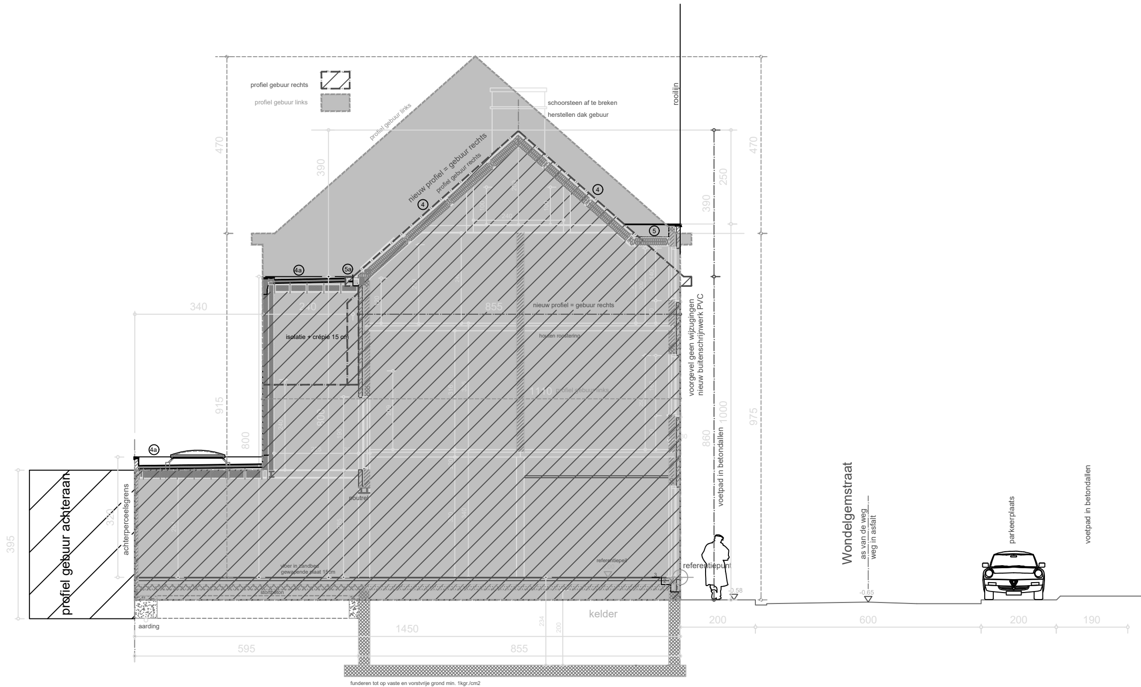
bestaande toestand zijgevel links / 1:100
