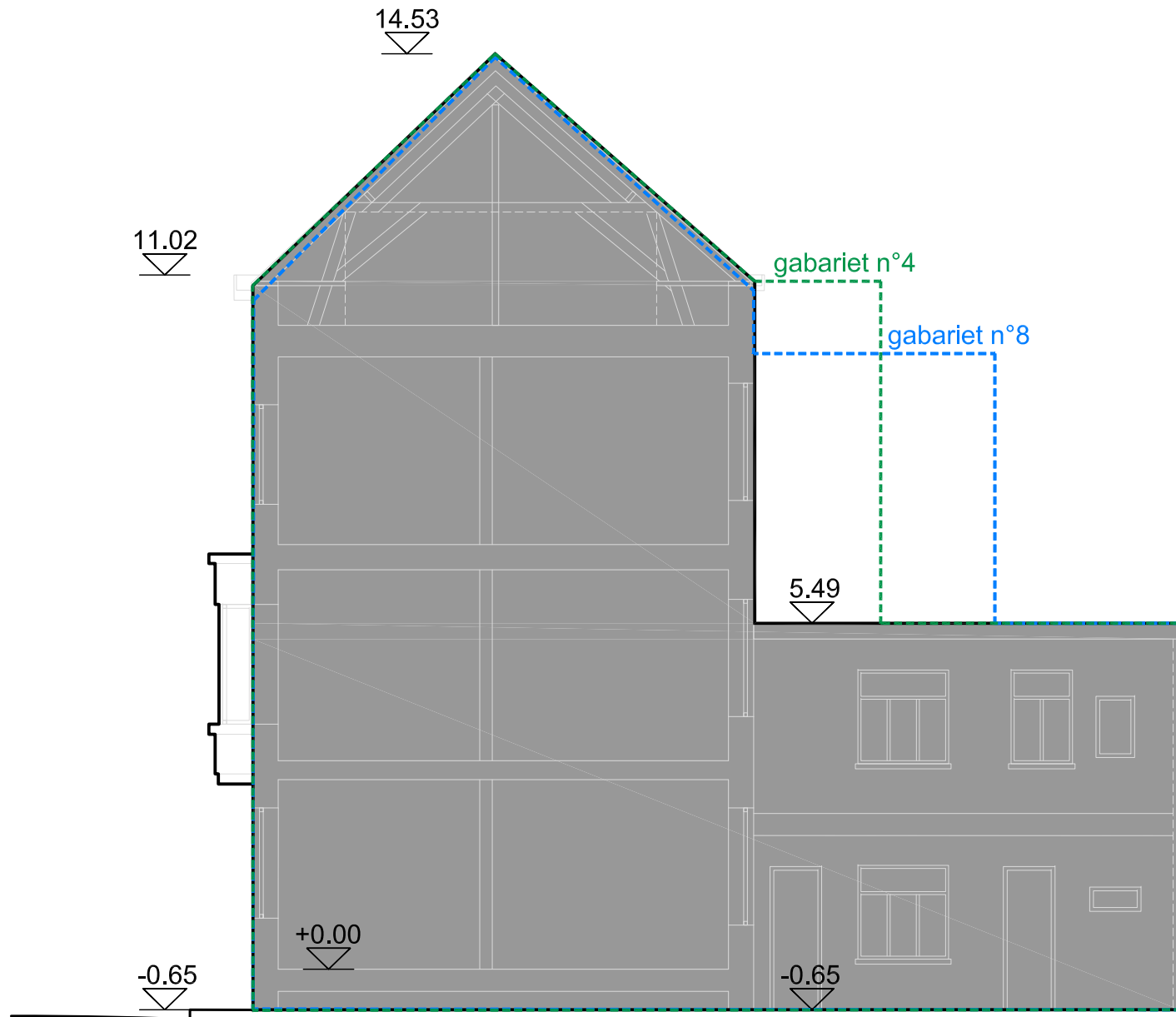
TERREINPROFIEL BESTAANDE TOESTAND
