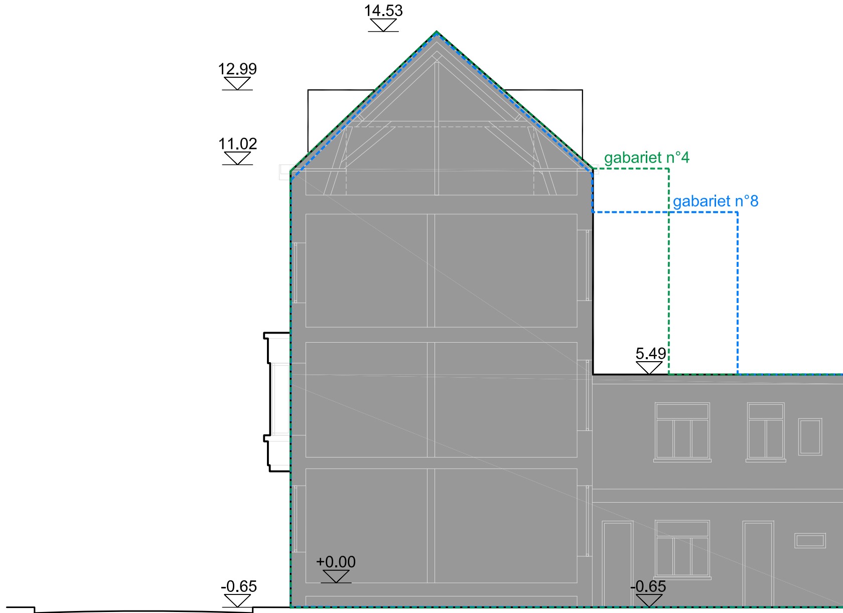
TERREINPROFIEL NIEUWE TOESTAND
