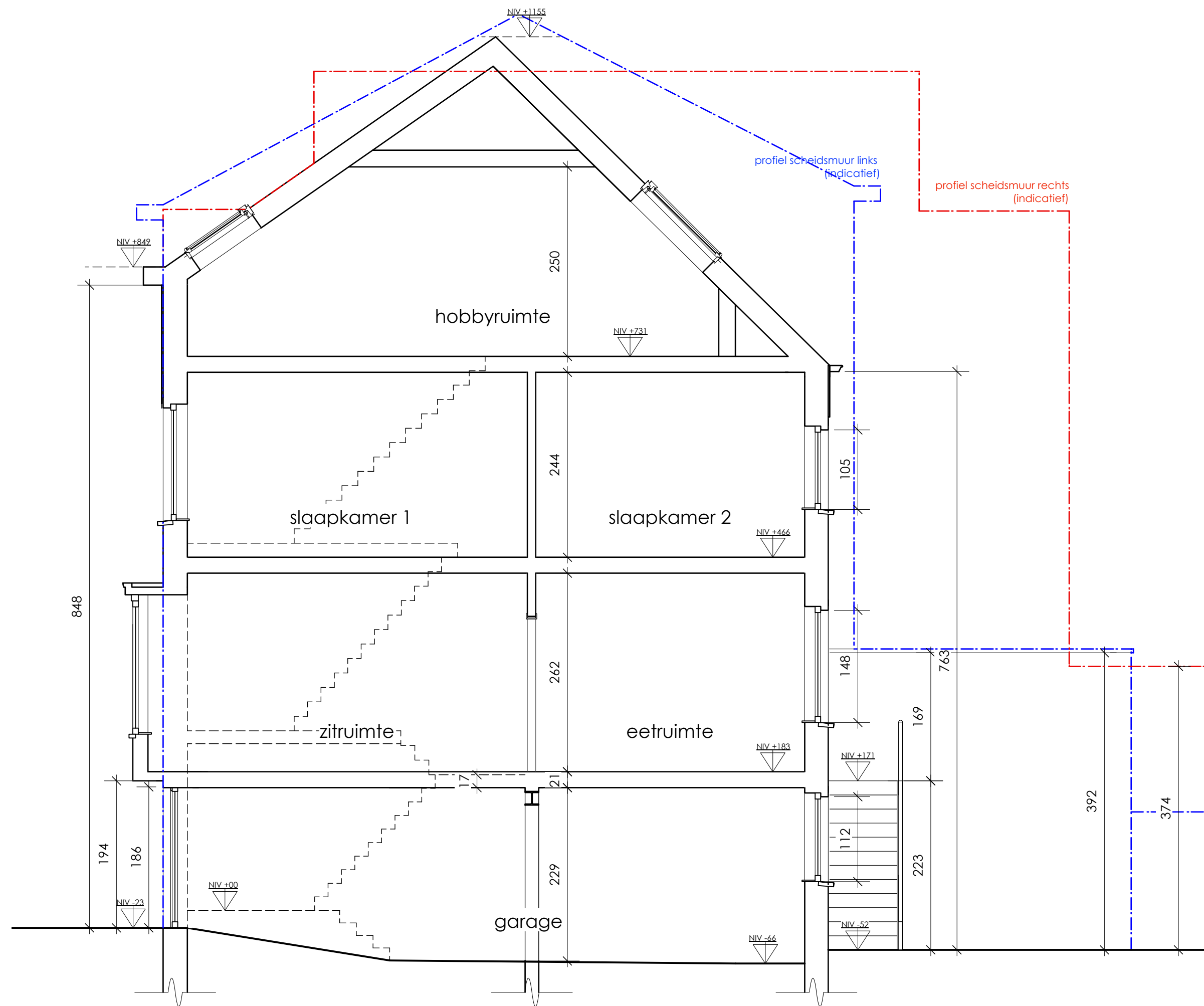
doorsnede AB
