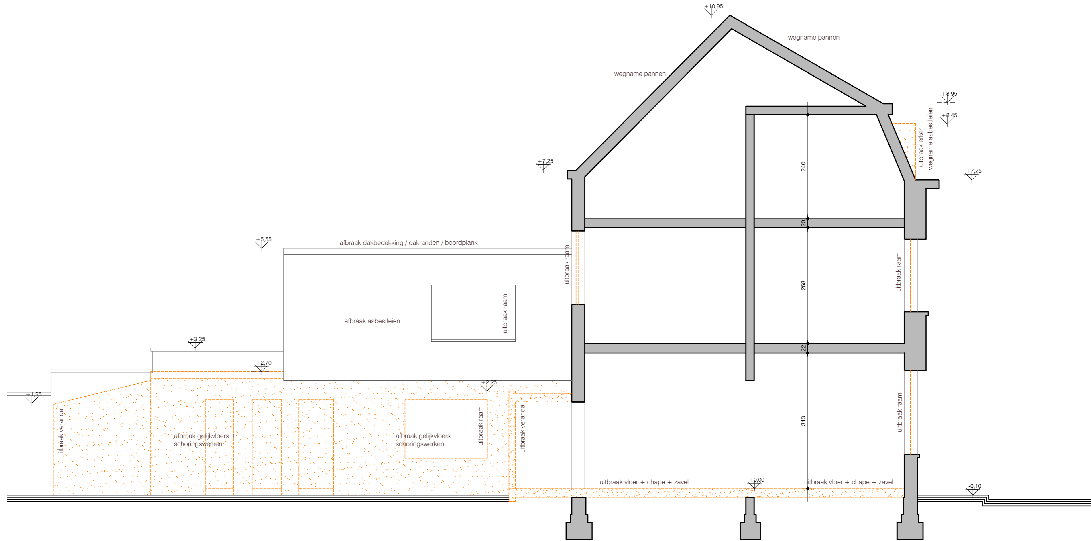
DOORSNEDE A-A bestaande toestand alle afmetingen zijn in cm schaal 1/50
