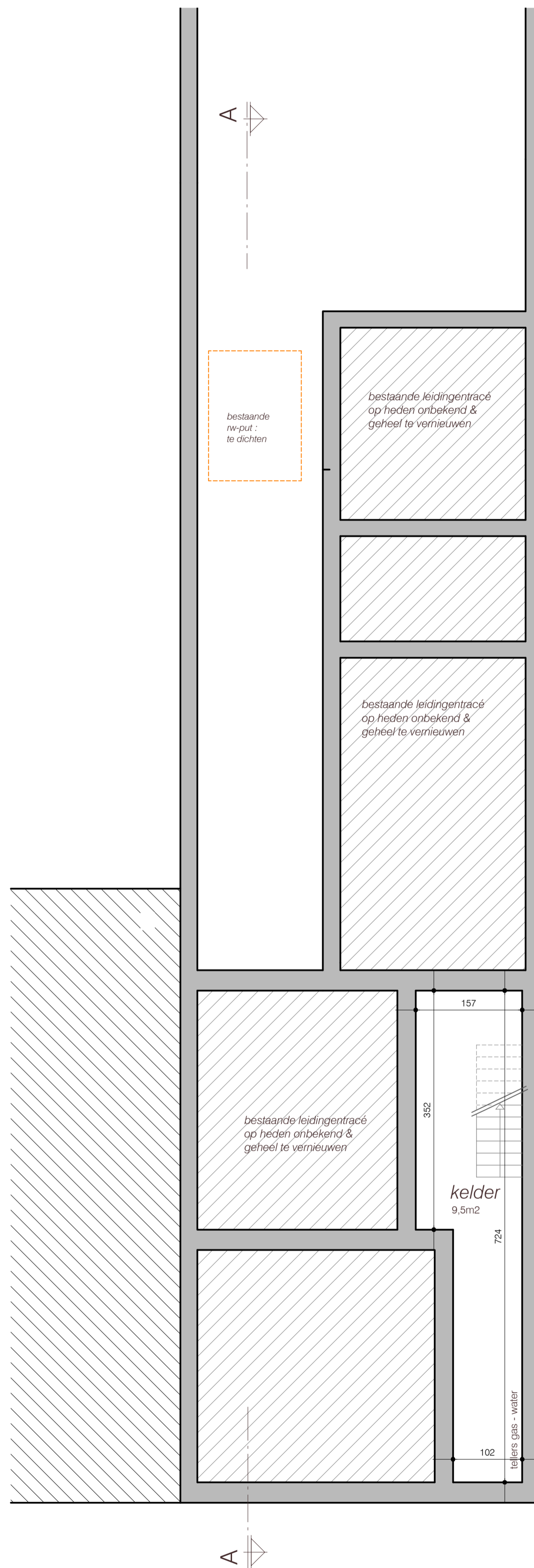
RIOLERING & FUNDERING bestaande toestand alle afmetingen zijn in cm schaal 1/50
