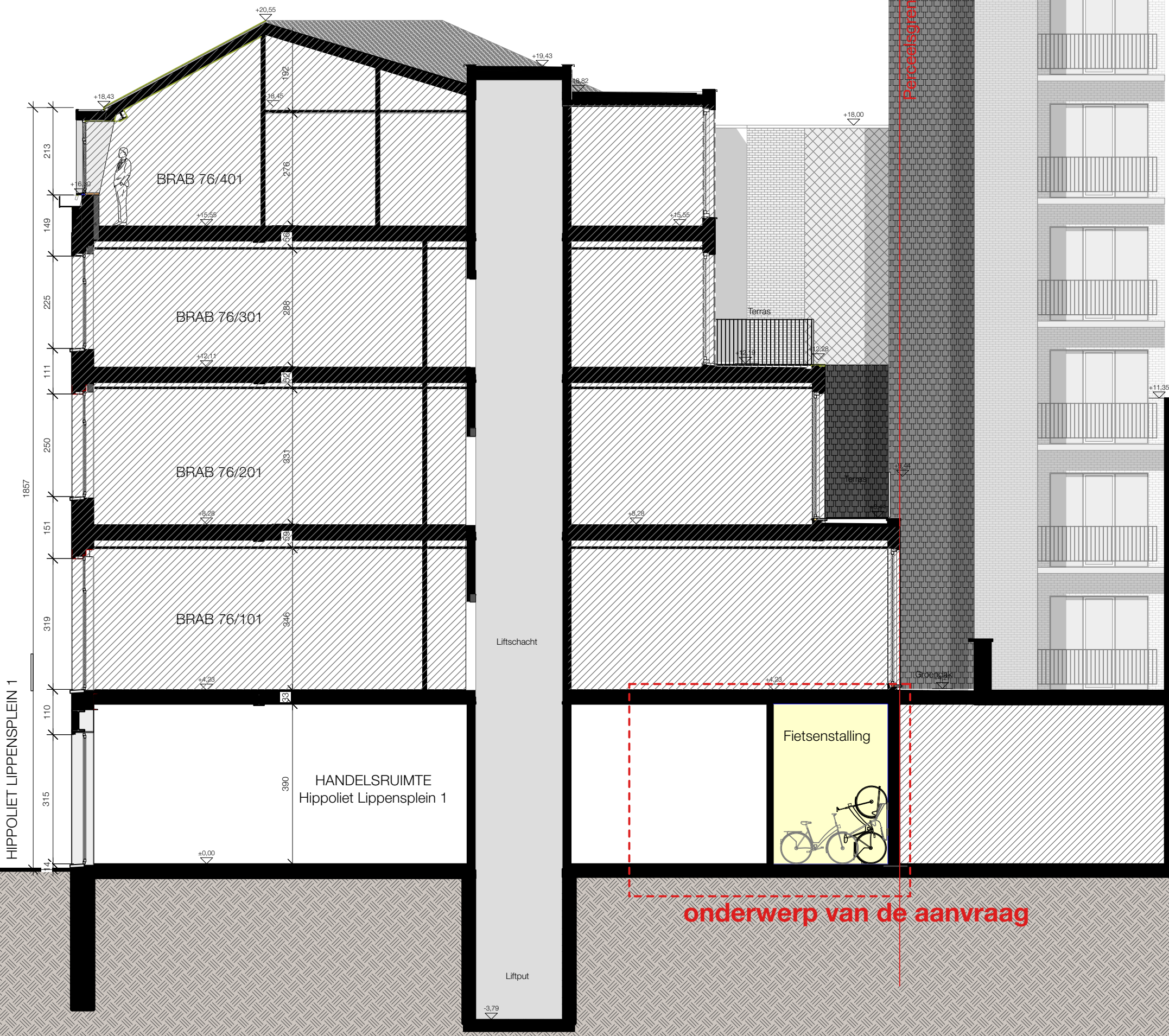
Snede B_ Bestaande toestand Schaal: 1:100
