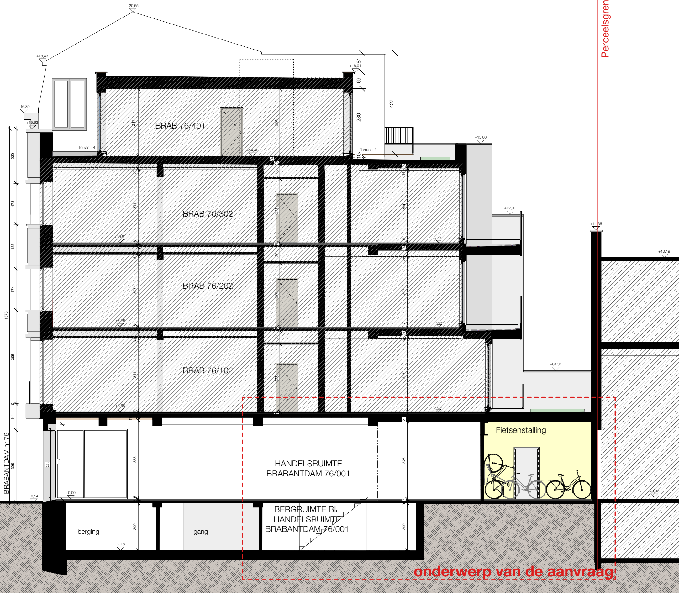
Snede A Bestaande toestand Schaal: 1:100
