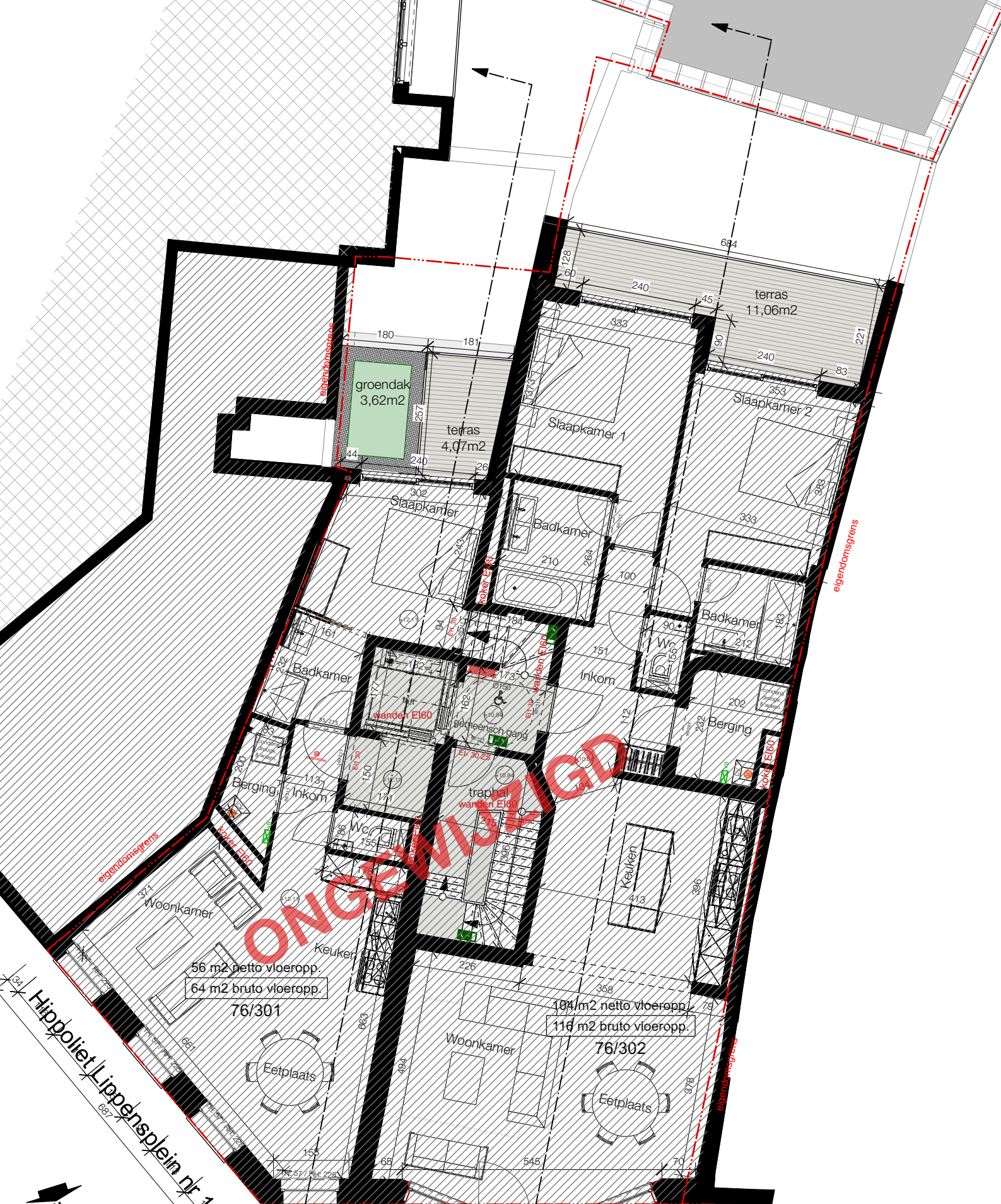
Brabantdam nr76 3e verdiep Nieuwe toestand Schaal: 1:100
