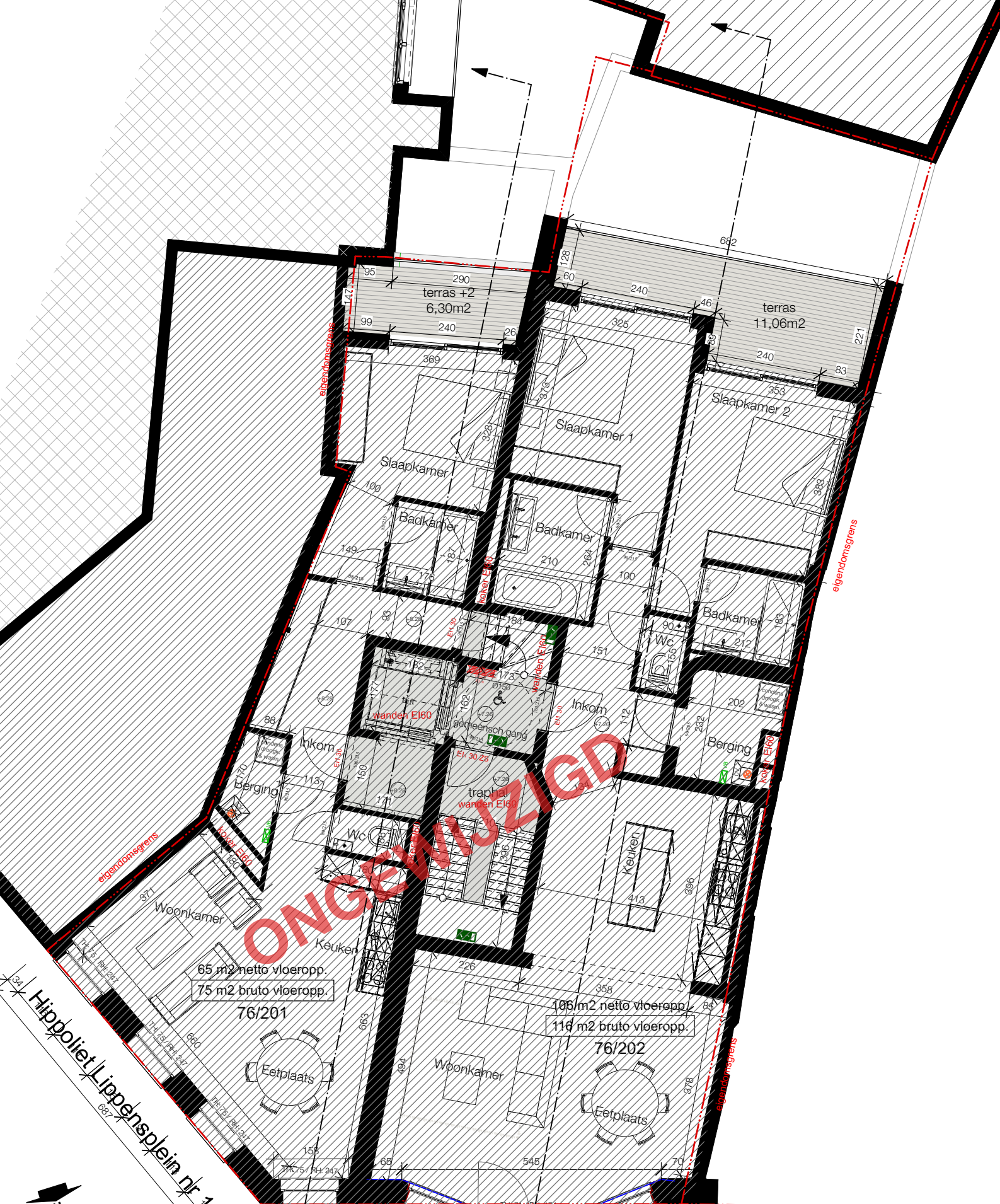
Brabantdam nr76 2e verdiep Nieuwe toestand Schaal: 1:100
