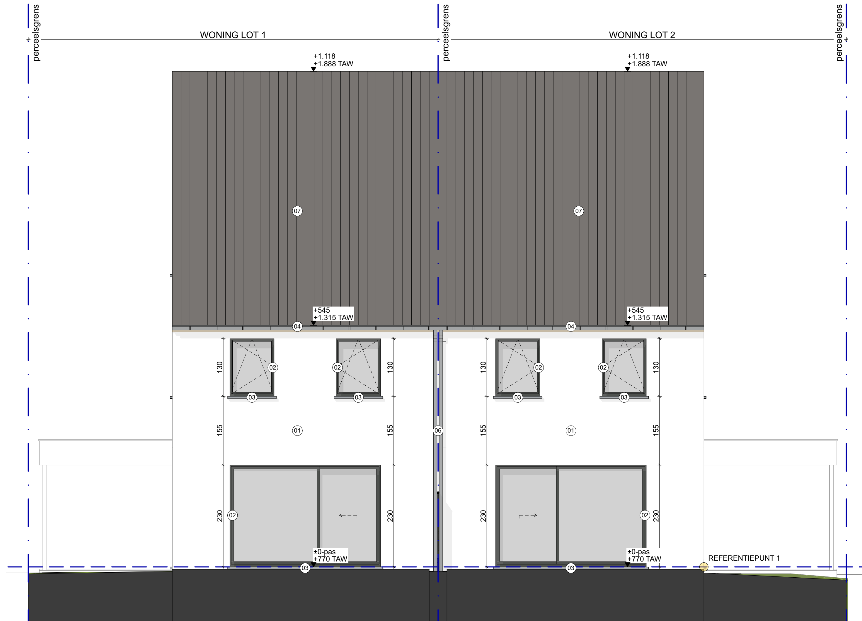
ACHTERGEVEL schaal 1:50 NIEUWE TOESTAND
