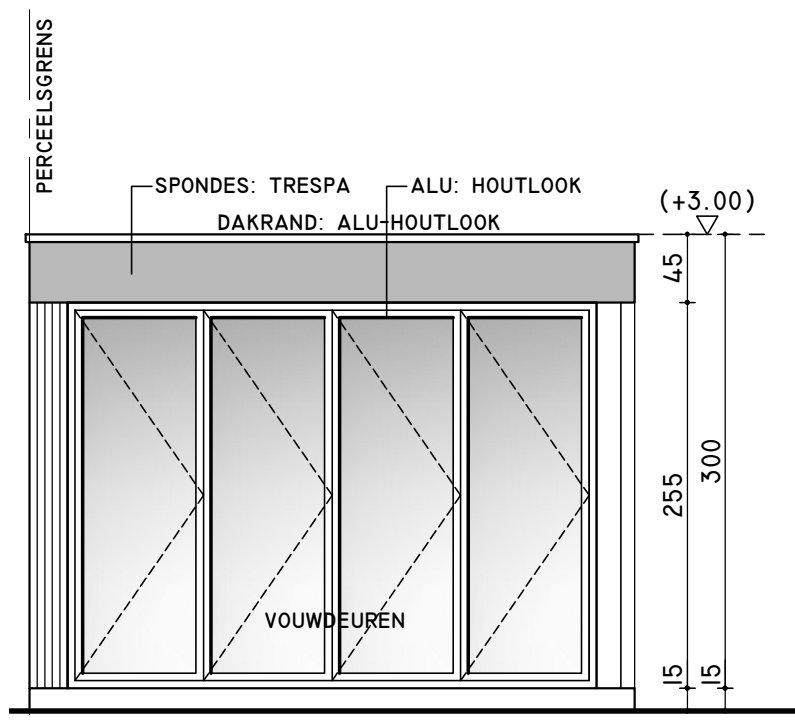
VOORGEVEL BIJGEBOUW
