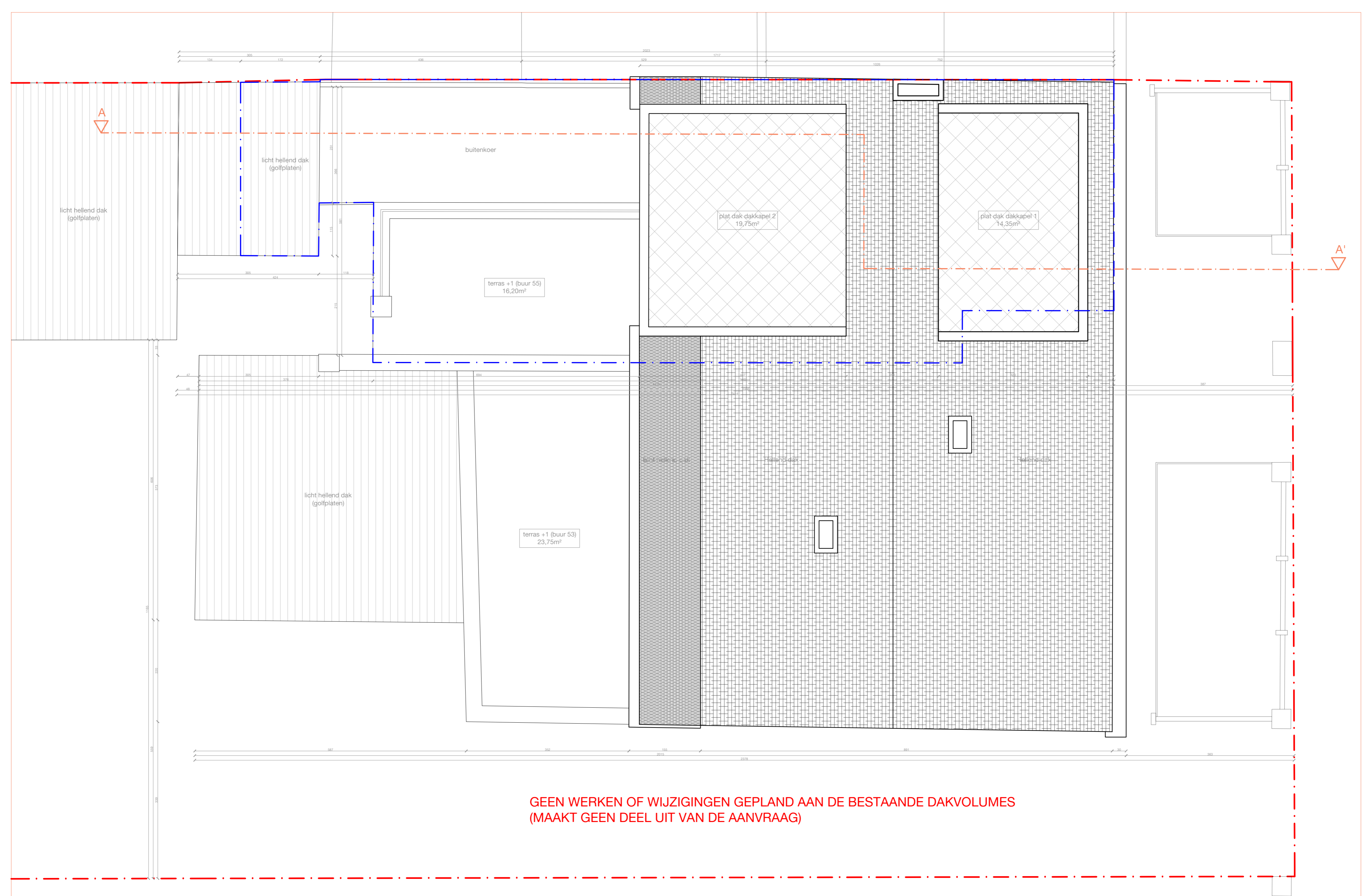
Dakenplan- bestaande situatie schaal 1:50
