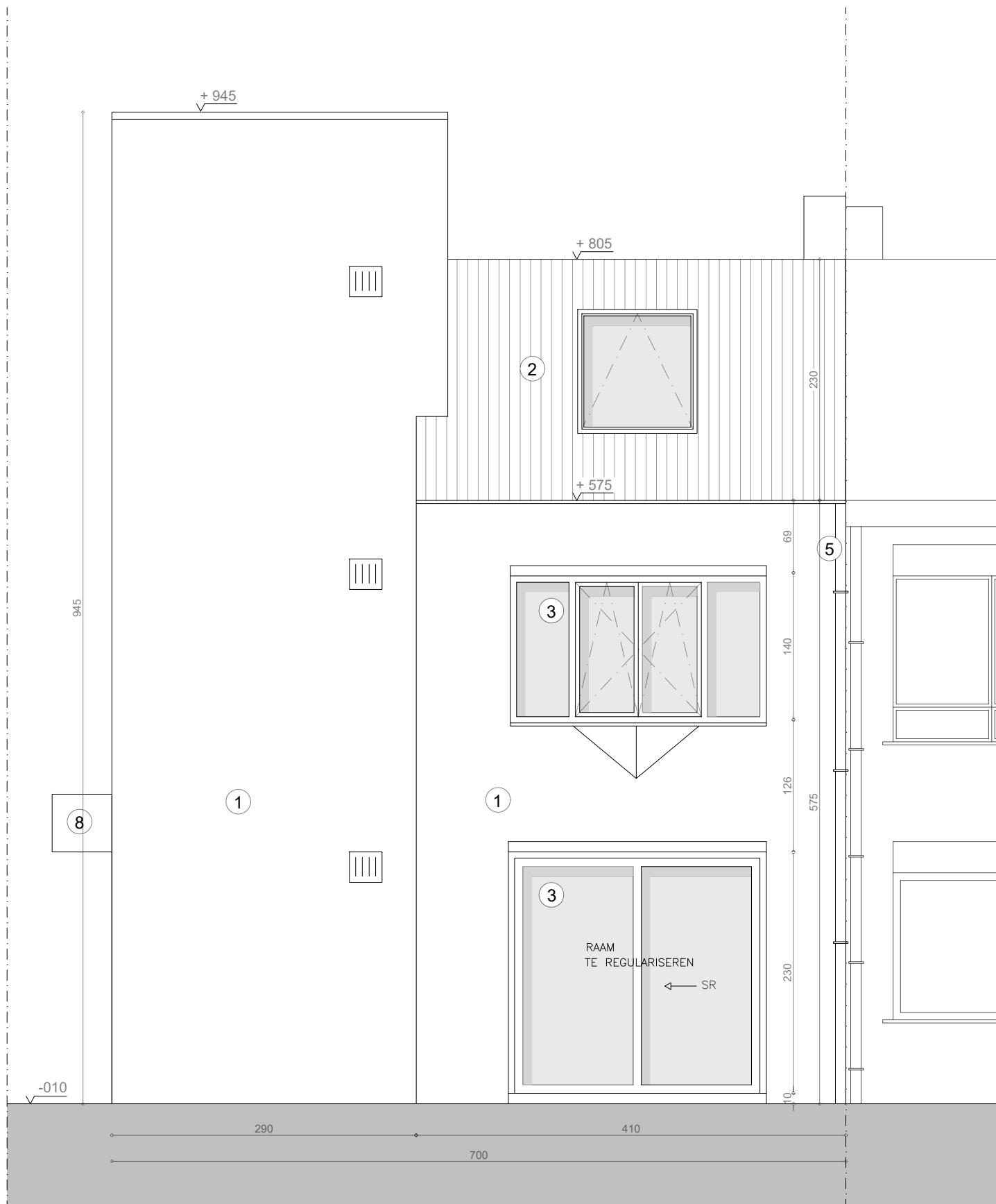
VOORGEVEL NIEUWE TOESTAND 1:50
