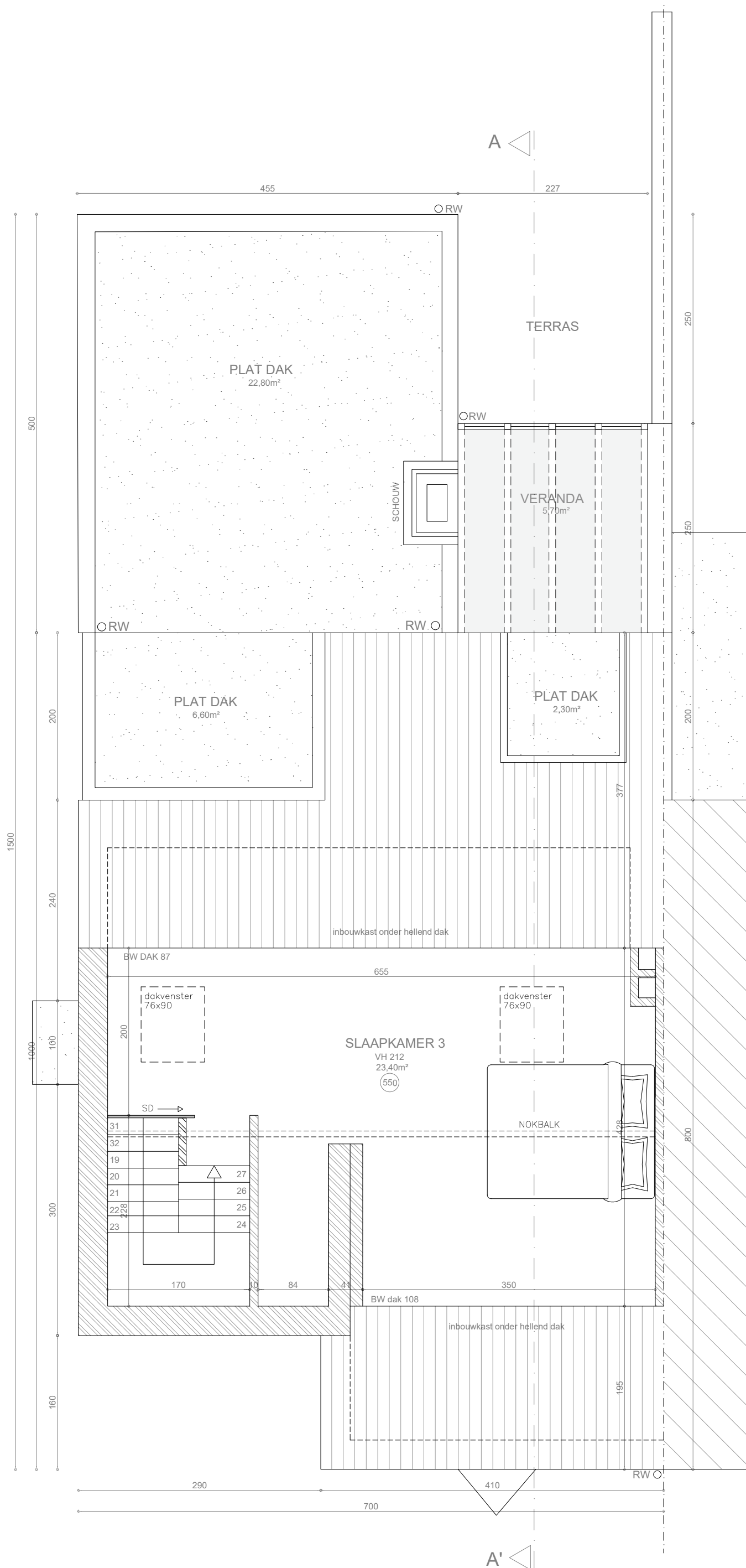
2E VERDIEPING BESTAANDE TOESTAND 1:50
