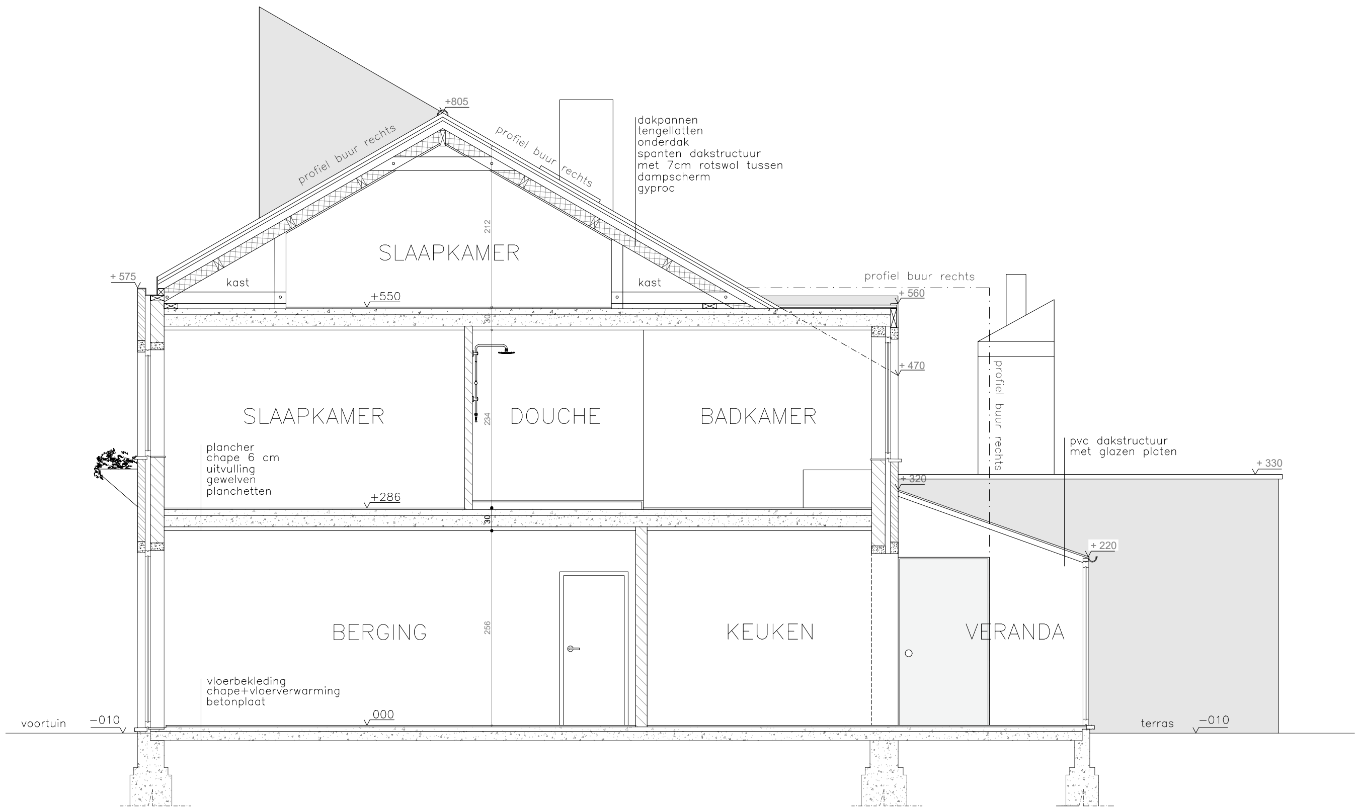
SNEDE BESTAANDE TOESTAND 1:50
