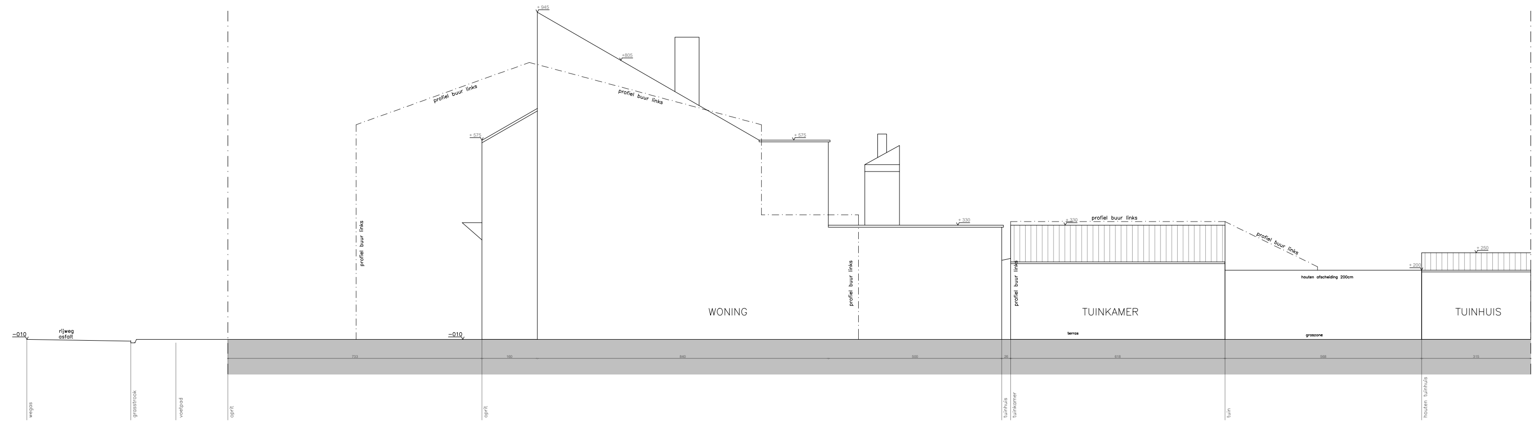
TERREINPROFIEL AA' BESTAANDE TOESTAND 1:100
