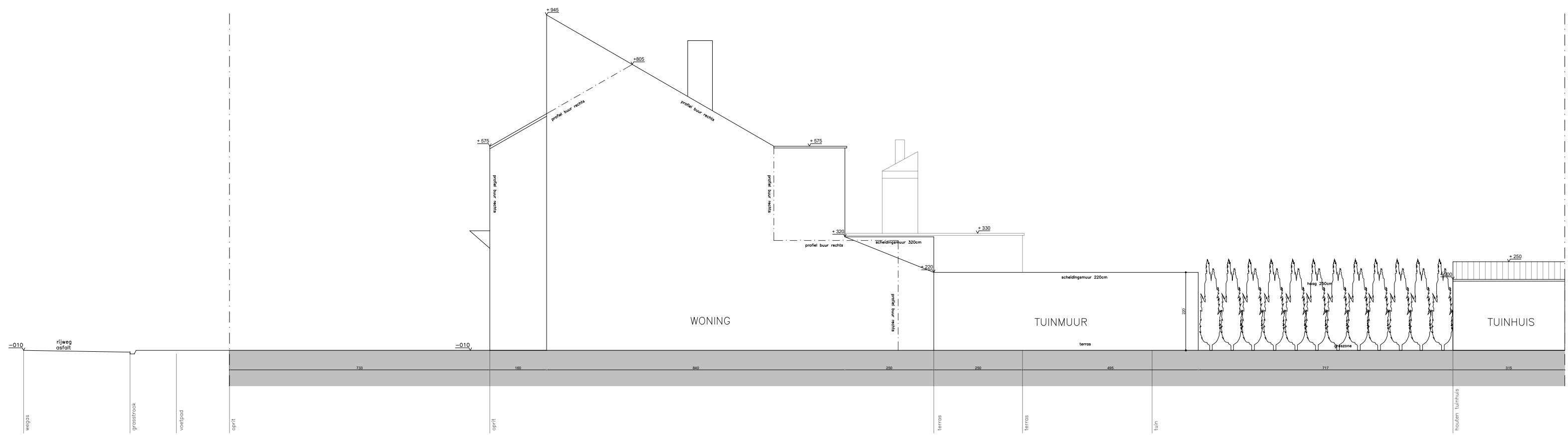
TERREINPROFIEL BB' BESTAANDE TOESTAND 1:100
