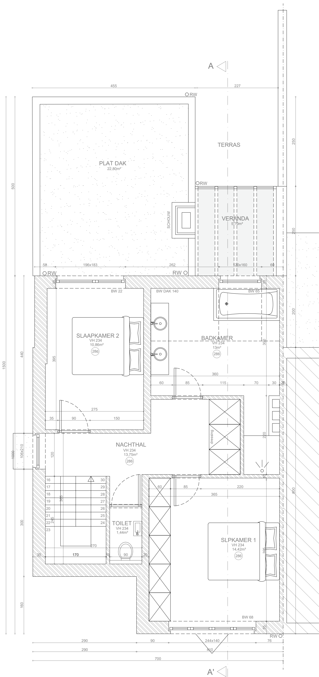
1E VERDIEPING BESTAANDE TOESTAND 1:50
