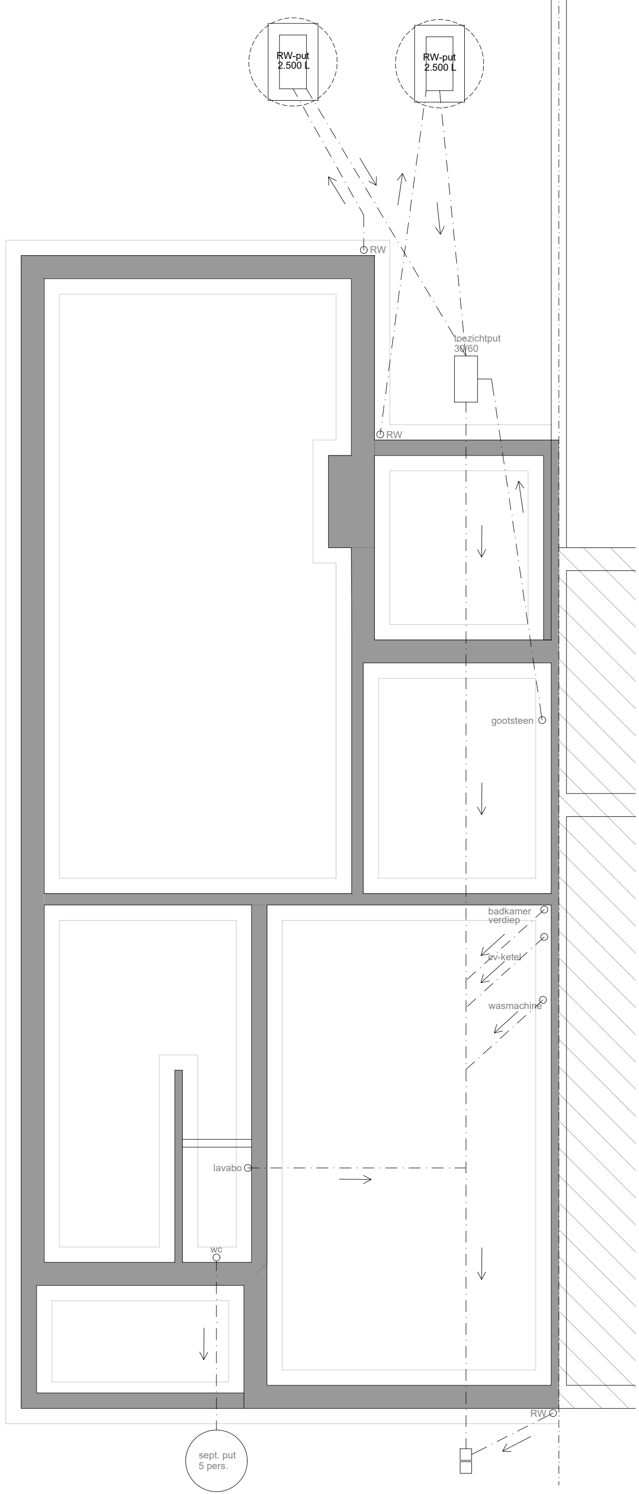
FUNDERINGSPLAN NIEUWE TOESTAND 1:50
