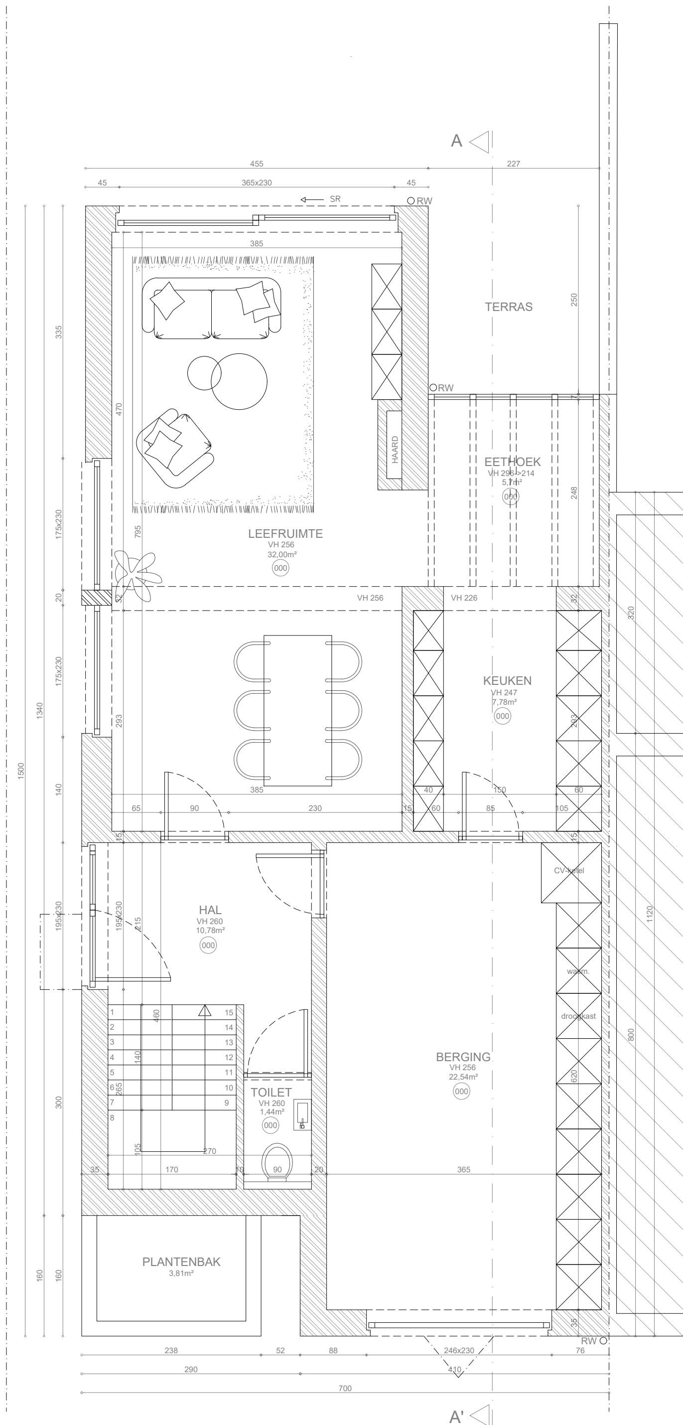
GRONDPLAN BESTAANDE TOESTAND 1:50
