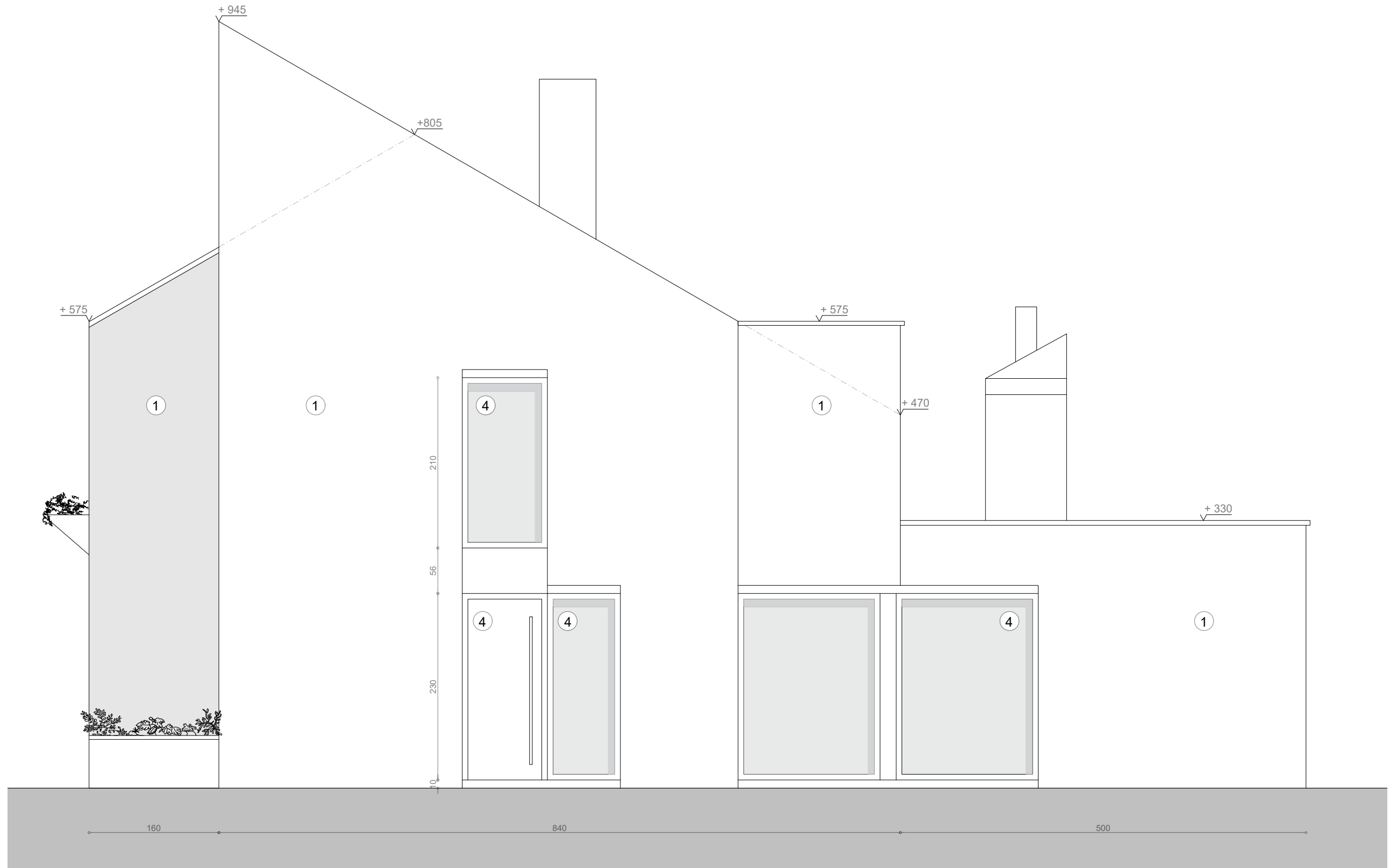
ZIJGEVEL BESTAANDE TOESTAND 1:50
