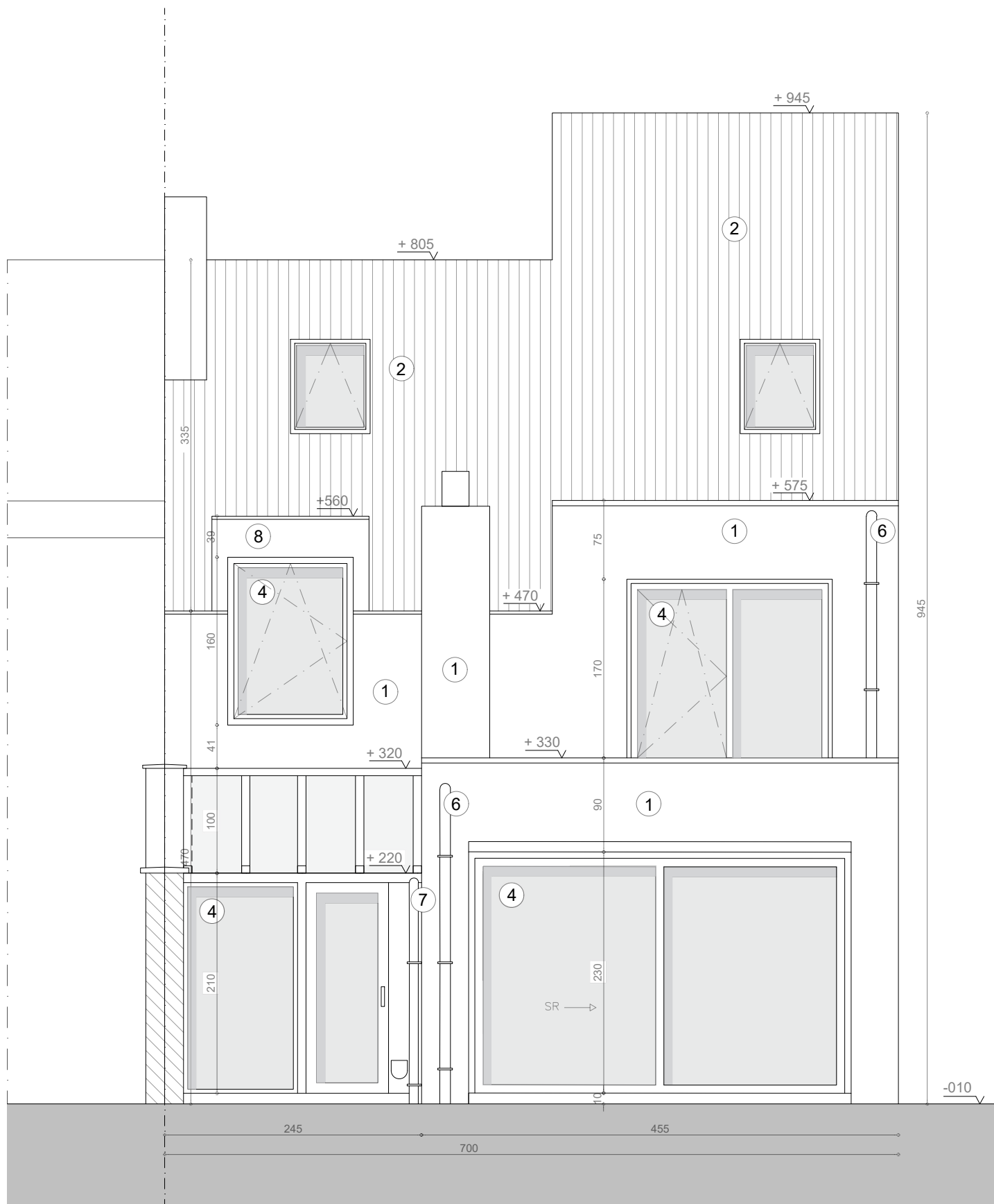
ACHTERGEVEL BESTAANDE TOESTAND 1:50
