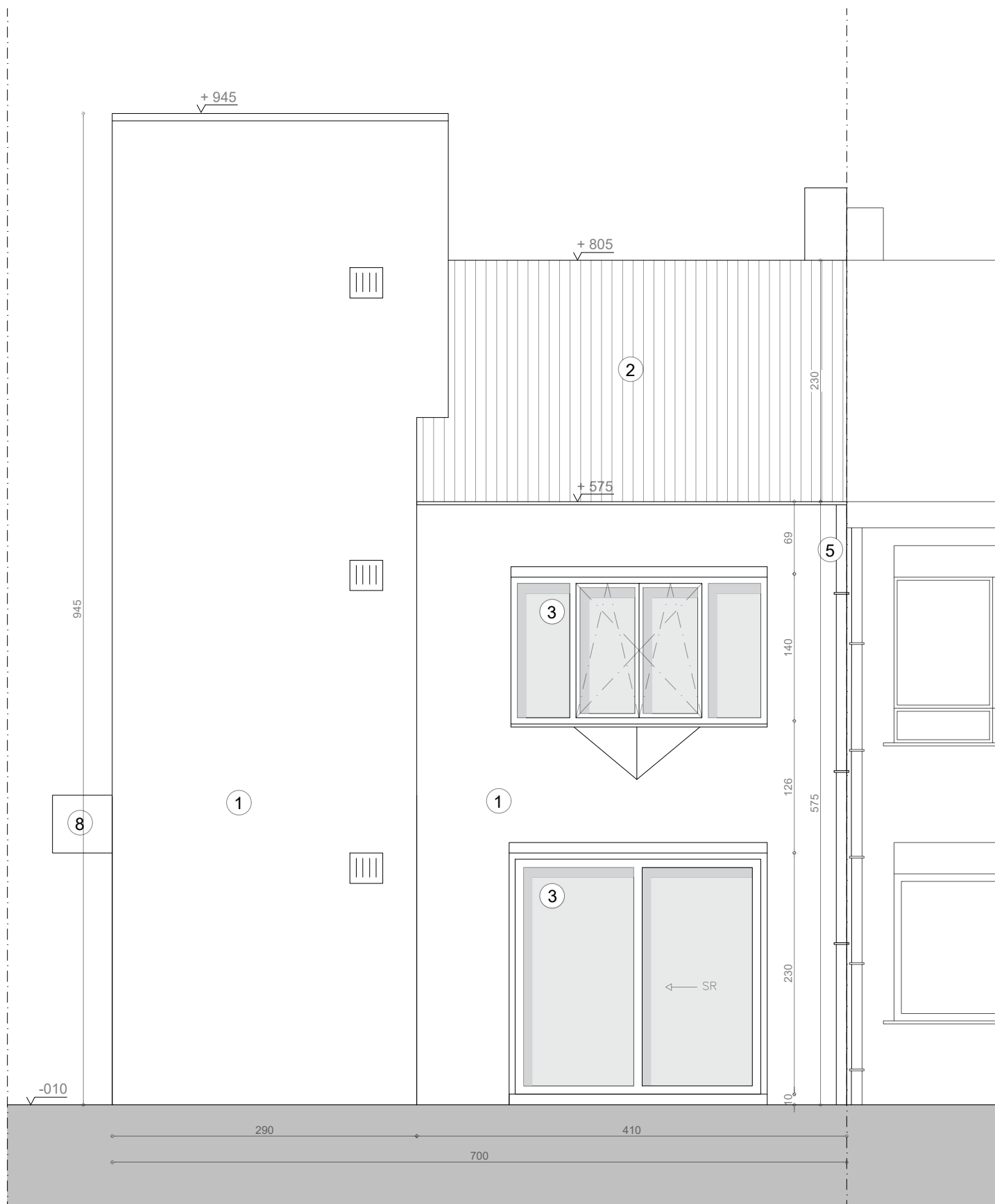
VOORGEVEL BESTAANDE TOESTAND 1:50
