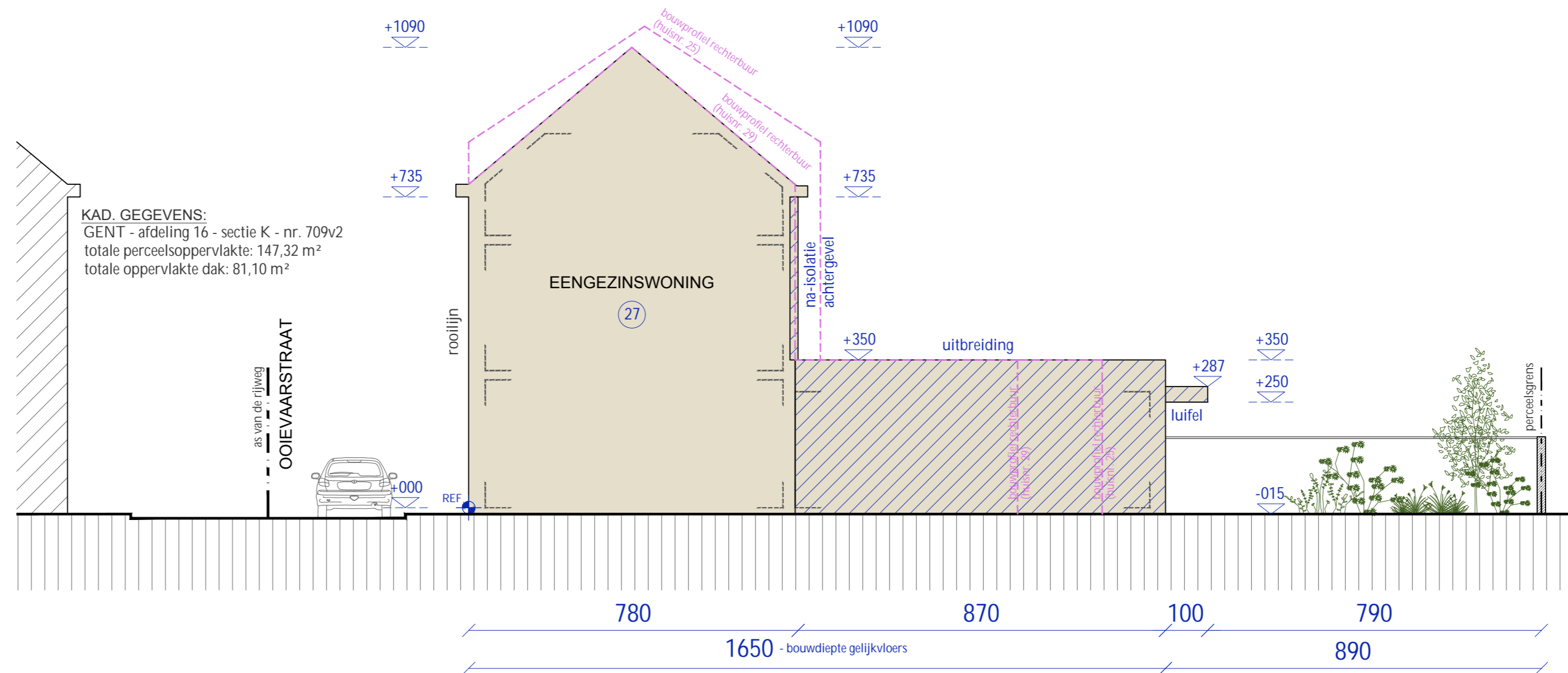
TERREINPROFIEL XX | nieuwe toestand
