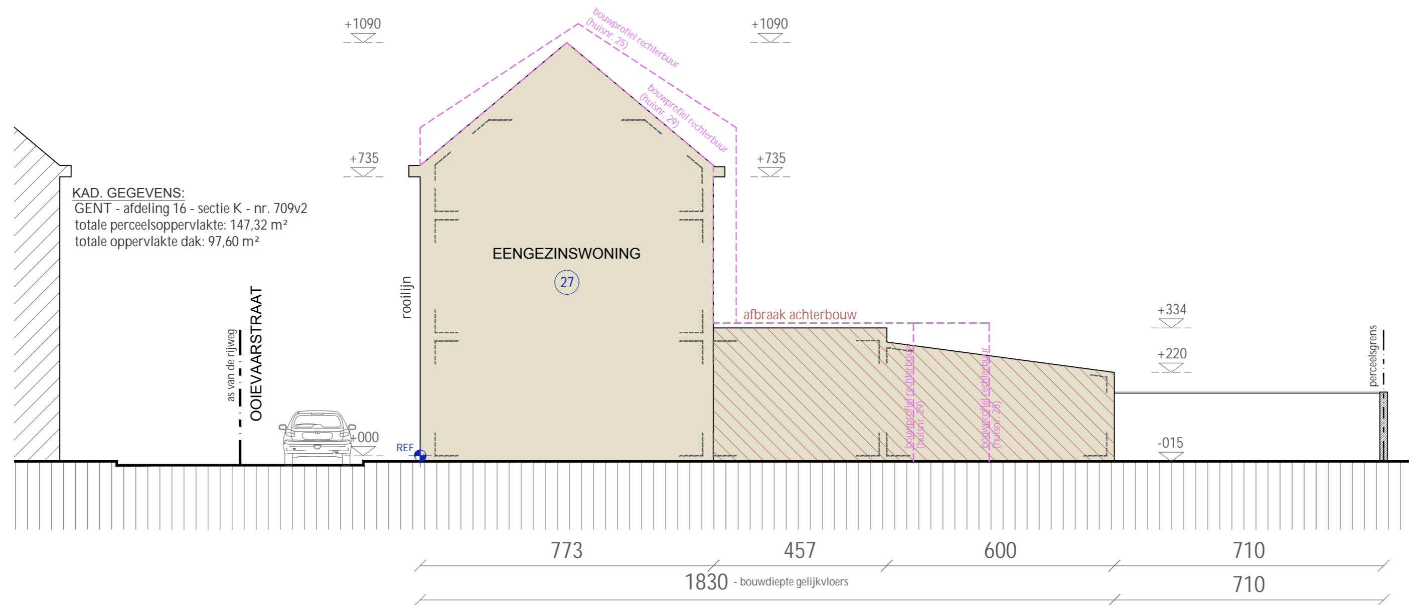
TERREINPROFIEL XX | bestaande toestand
