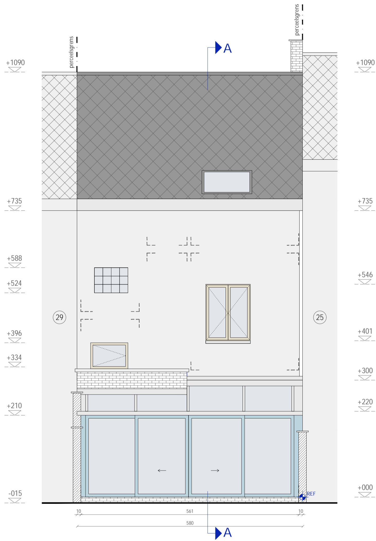
ACHTERGEVEL | bestaande toestand
