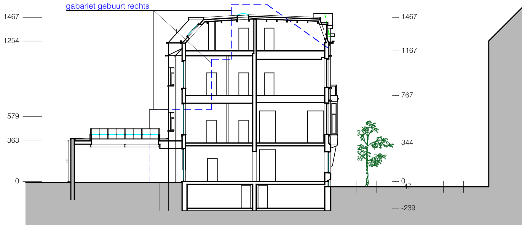
terreinprofiel 2 - vergunde toestand
