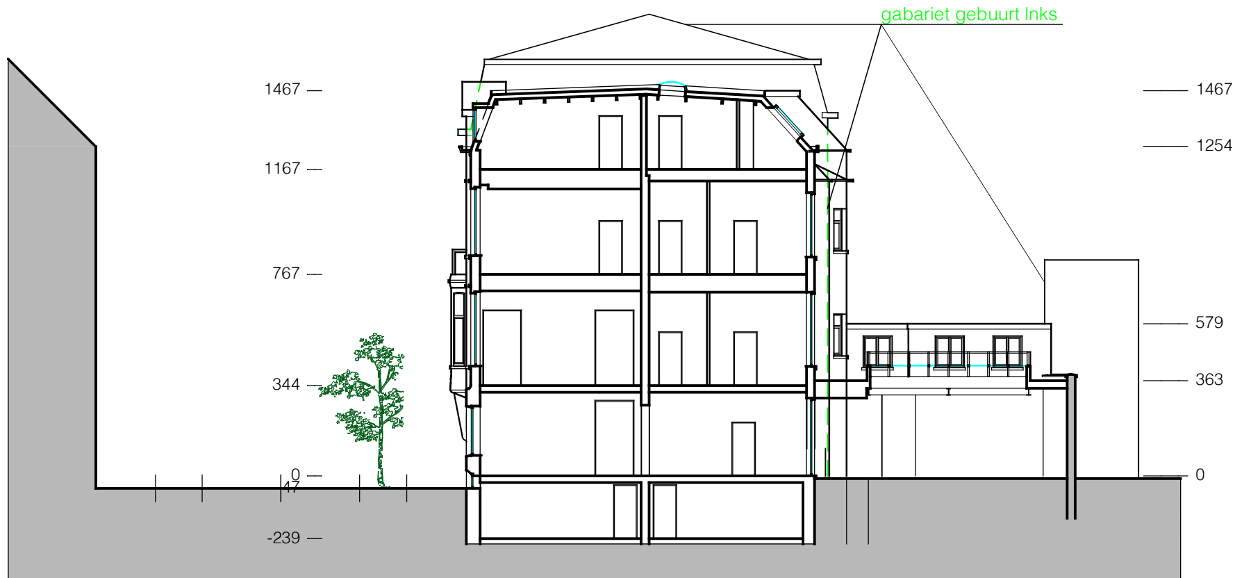
terreinprofiel 1 - huidige toestand
