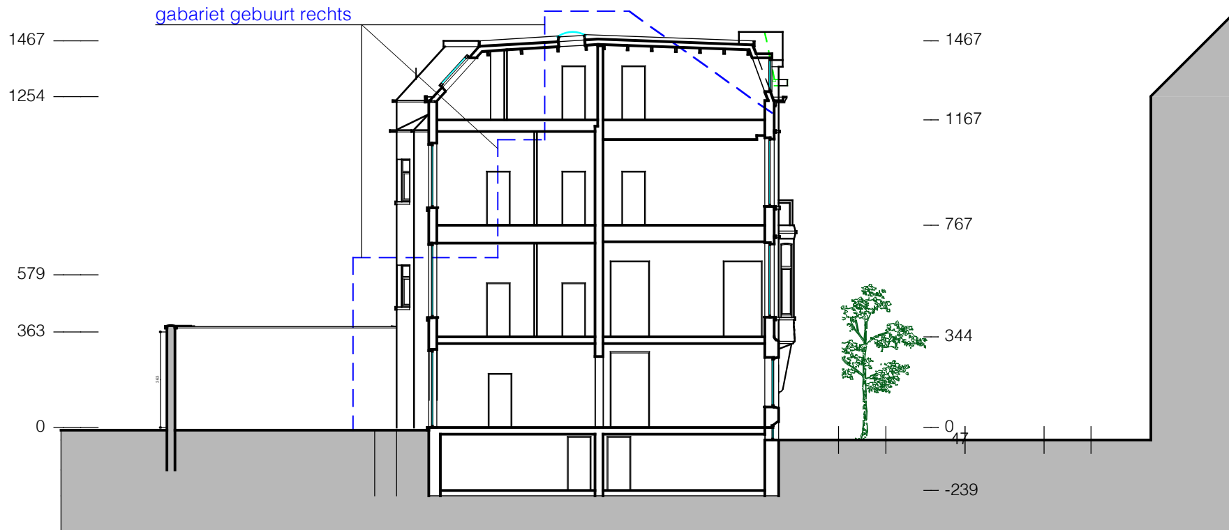
terreinprofiel 2 - oorspronkelijke toestand
