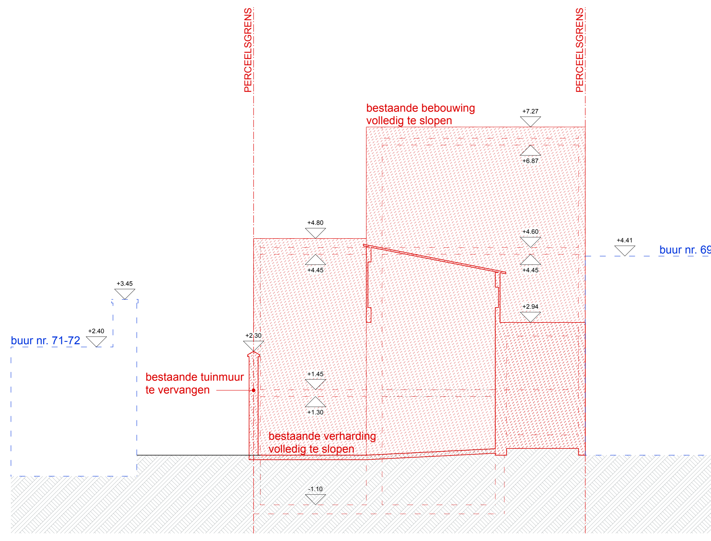
Snede BB
