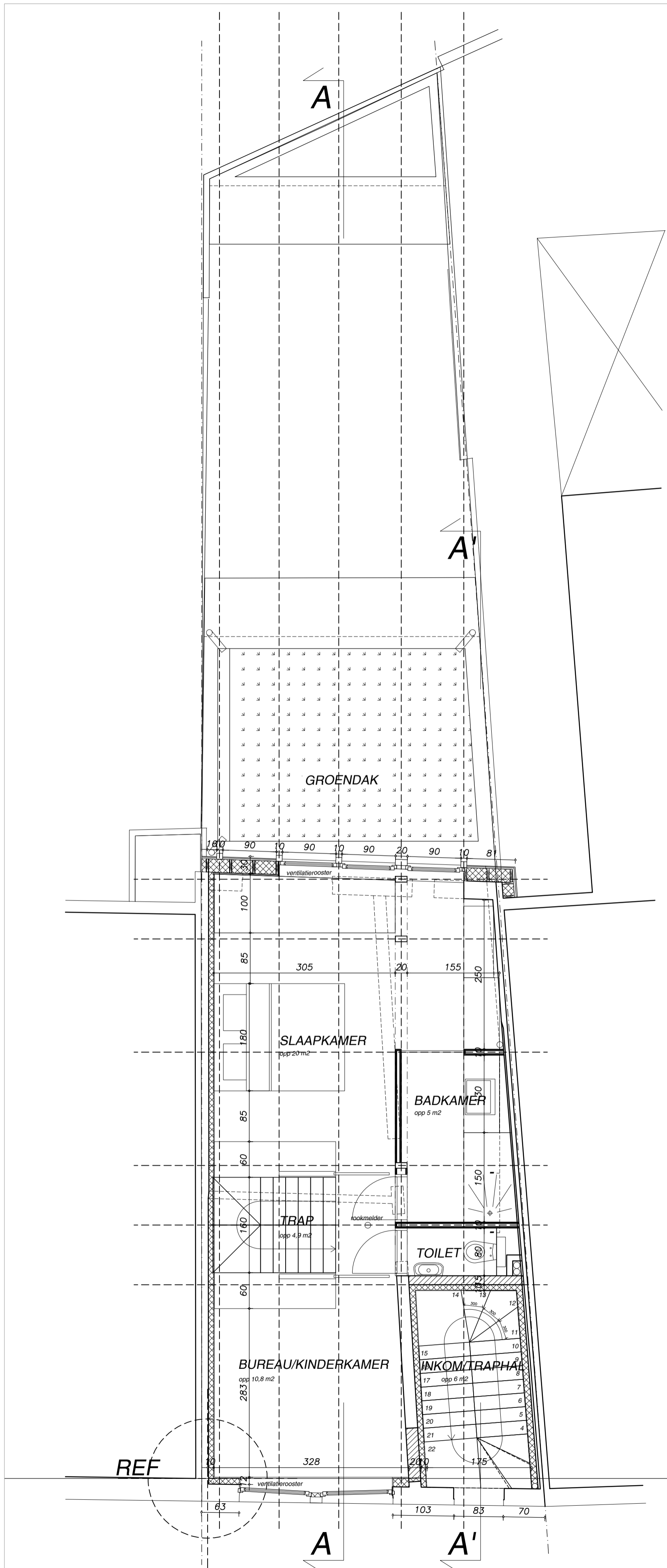
VERDIEP+1 PLAN 1/50 vergunde toestand
