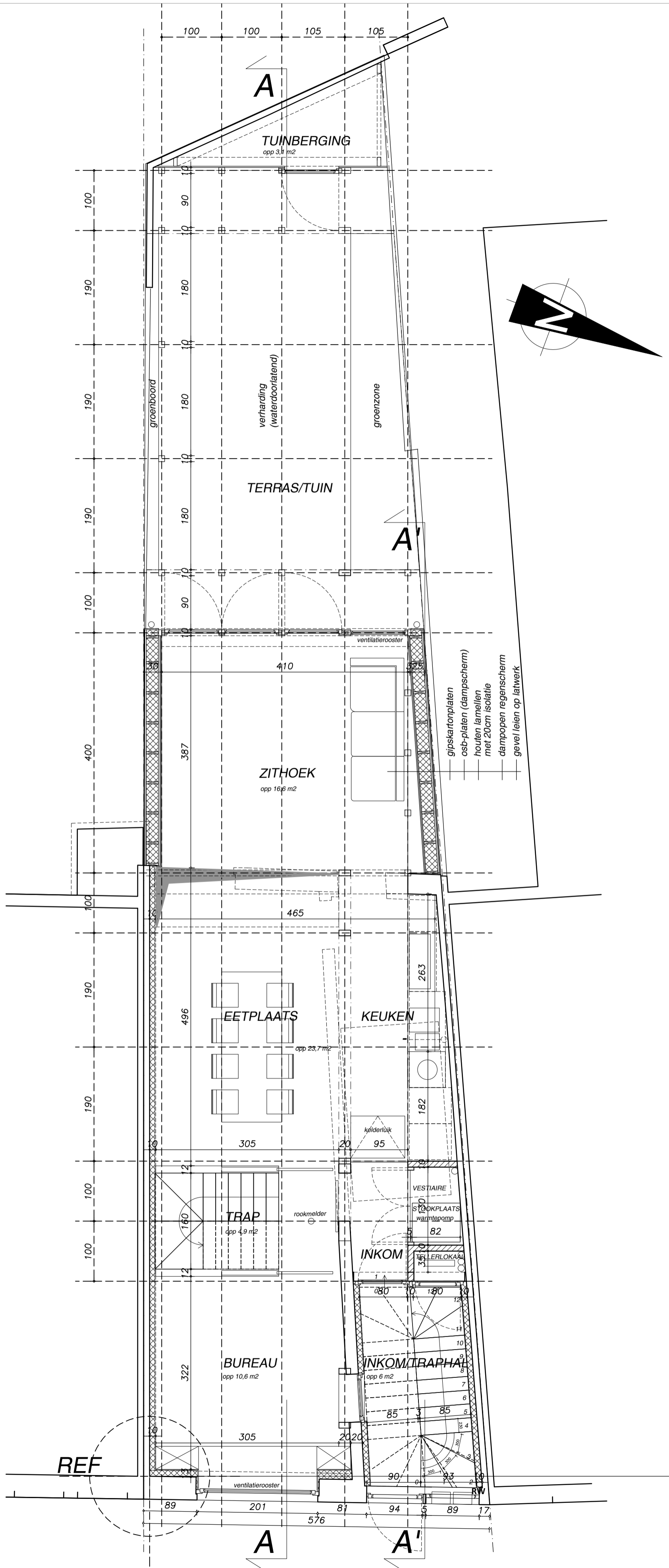
GRONDPLAN vergunde toestand
