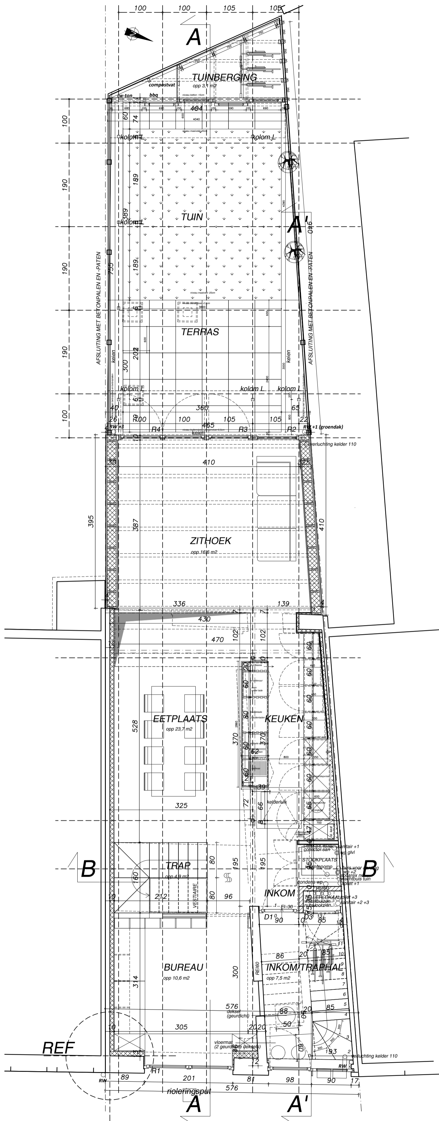
GRONDPLAN 1/50 0 2.5m
