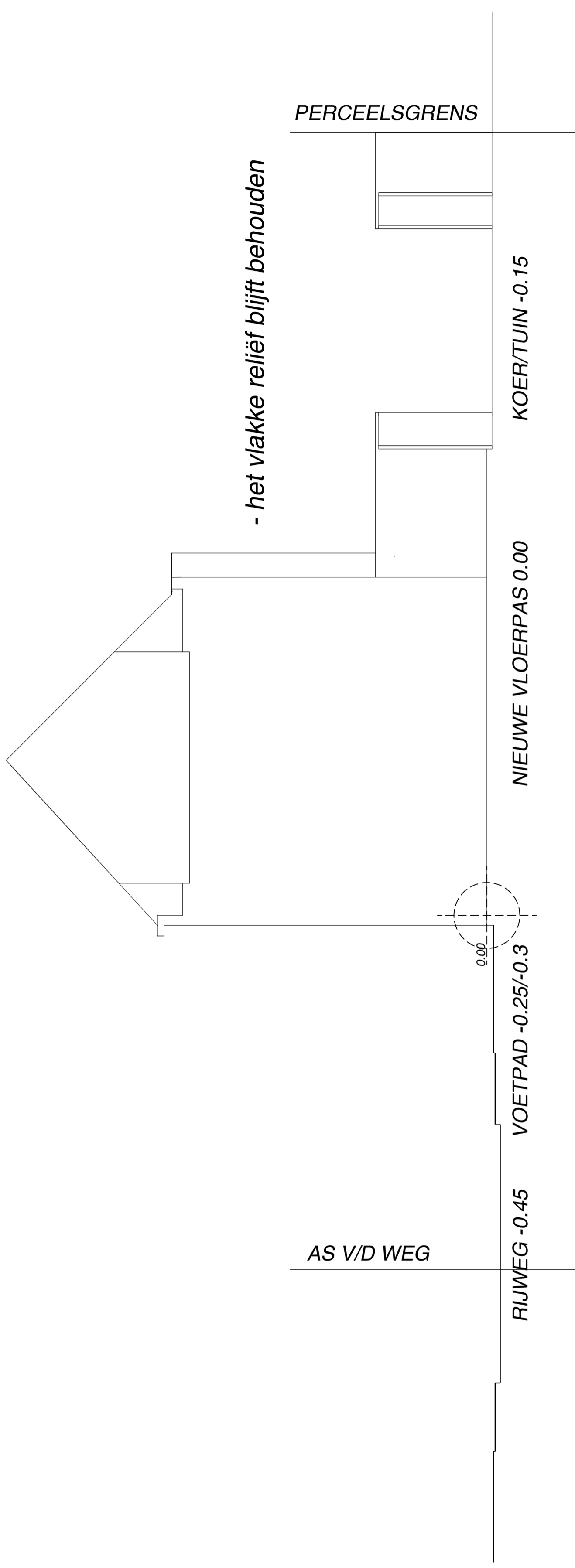
TERREINPROFIEL XX 1/100 vergunde toestand = bestaande toestand = nieuwe situatie
