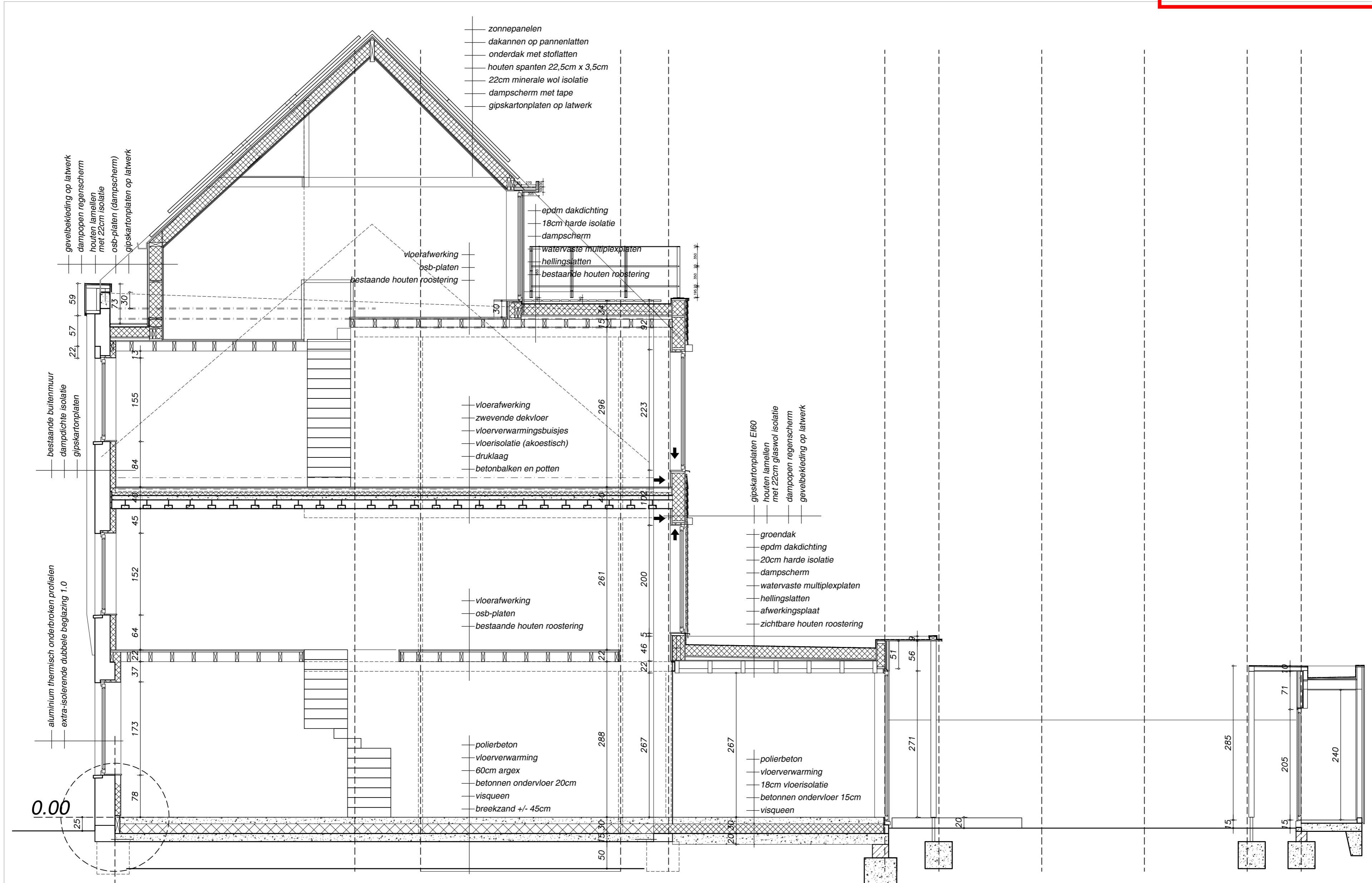
DOORSNEDE AA 1/50 0 2.5m
