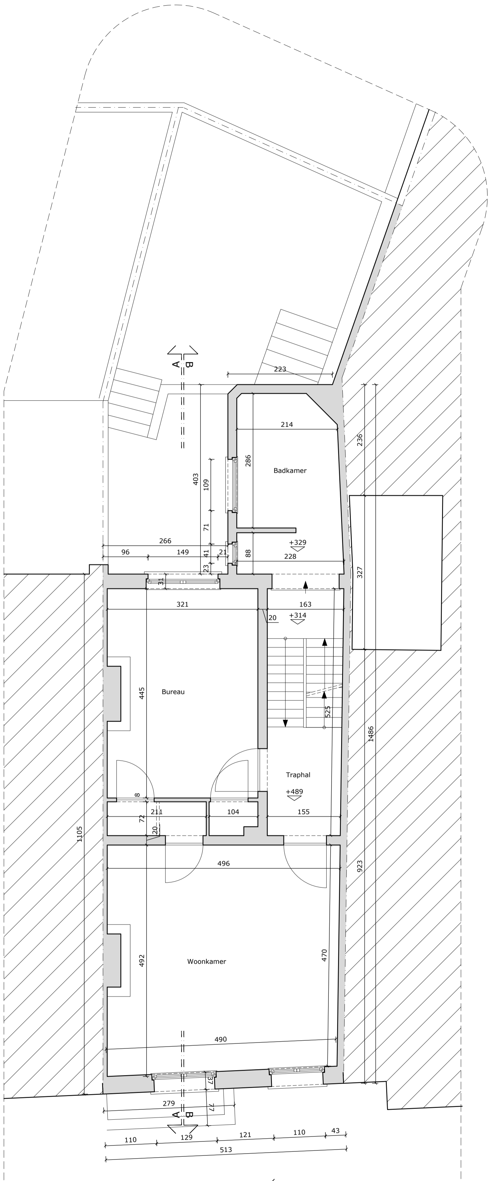
PLAN VERDIEPING 1 AFMETINGEN OP PLAN IN CENTIMETER bestaande toestand - 1/50
