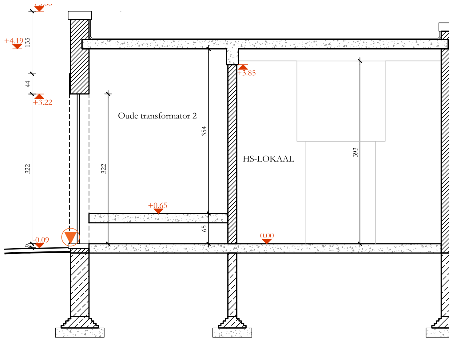
SNEDE B-B BESTAANDE TOESTAND OP SCHAAL 1 / 50
