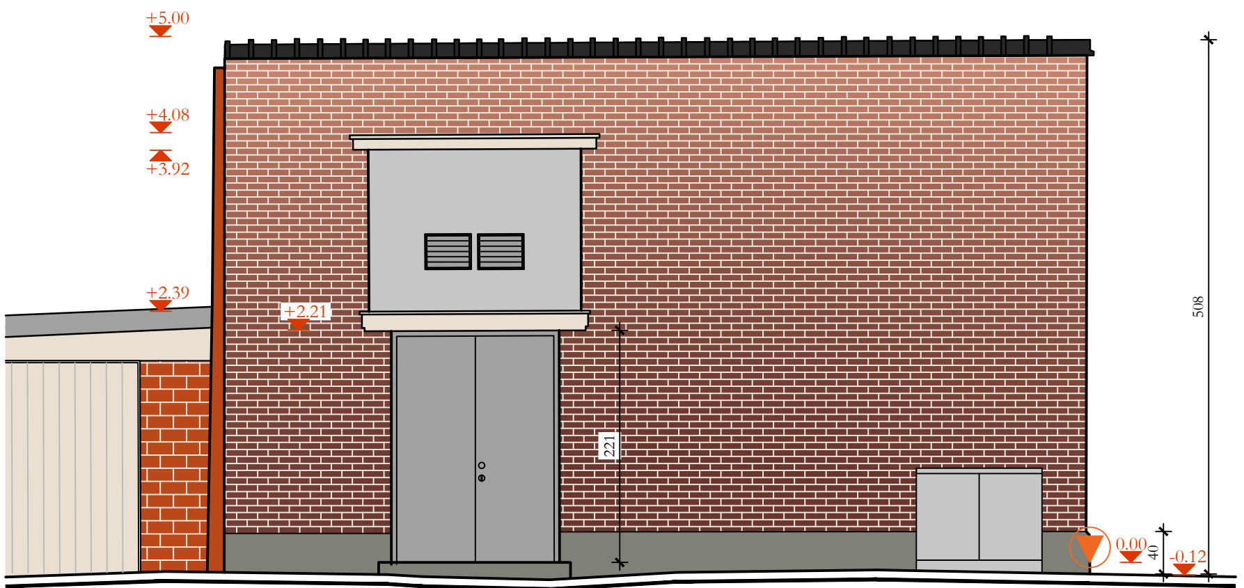
ZIJGEVEL LINKS BESTAANDE TOESTAND OP SCHAAL 1 / 50
