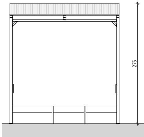
ACHTERAANZICHT
