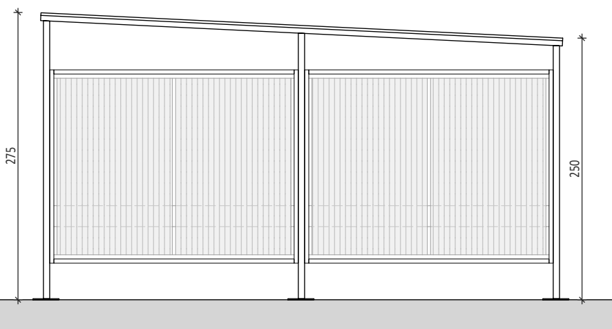
ZIJ-AANZICHT RECHTS
