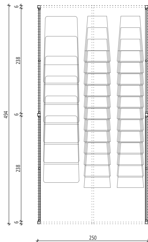
GRONDPLAN
