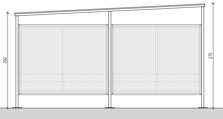
ZIJ-AANZICHT LINKS
